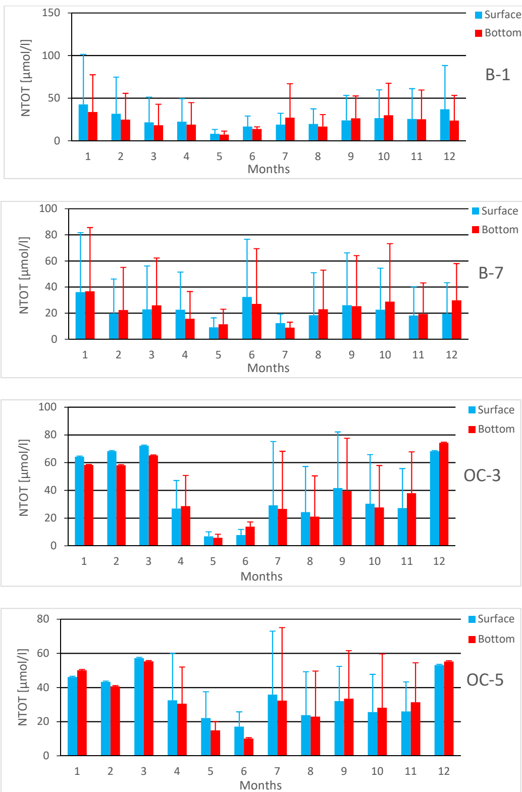
Slika 2.114: Prosječne mjesečne koncentracije ukupnog azota sa standardnim devijacijama za površinski i pridneni sloj vodenog stuba za lokacije B1, B7, OC3 i OC5 tokom perioda 2009-2019. Izvor podataka: IBM-Kotor, CETI-Podgorica
