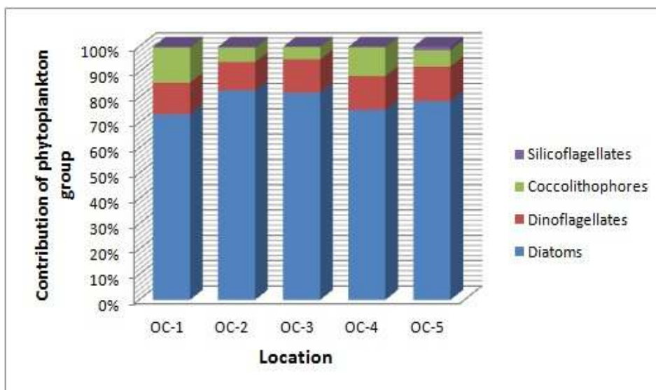
Slika 2.20: Udio taksonomskih grupa mikroplanktona u ukupnoj brojnosti fitoplanktona na lokalitetima Bokotorskog zaliva I u priobalnom dijelu otvorenog mora u periodu 2009-2019. godine
