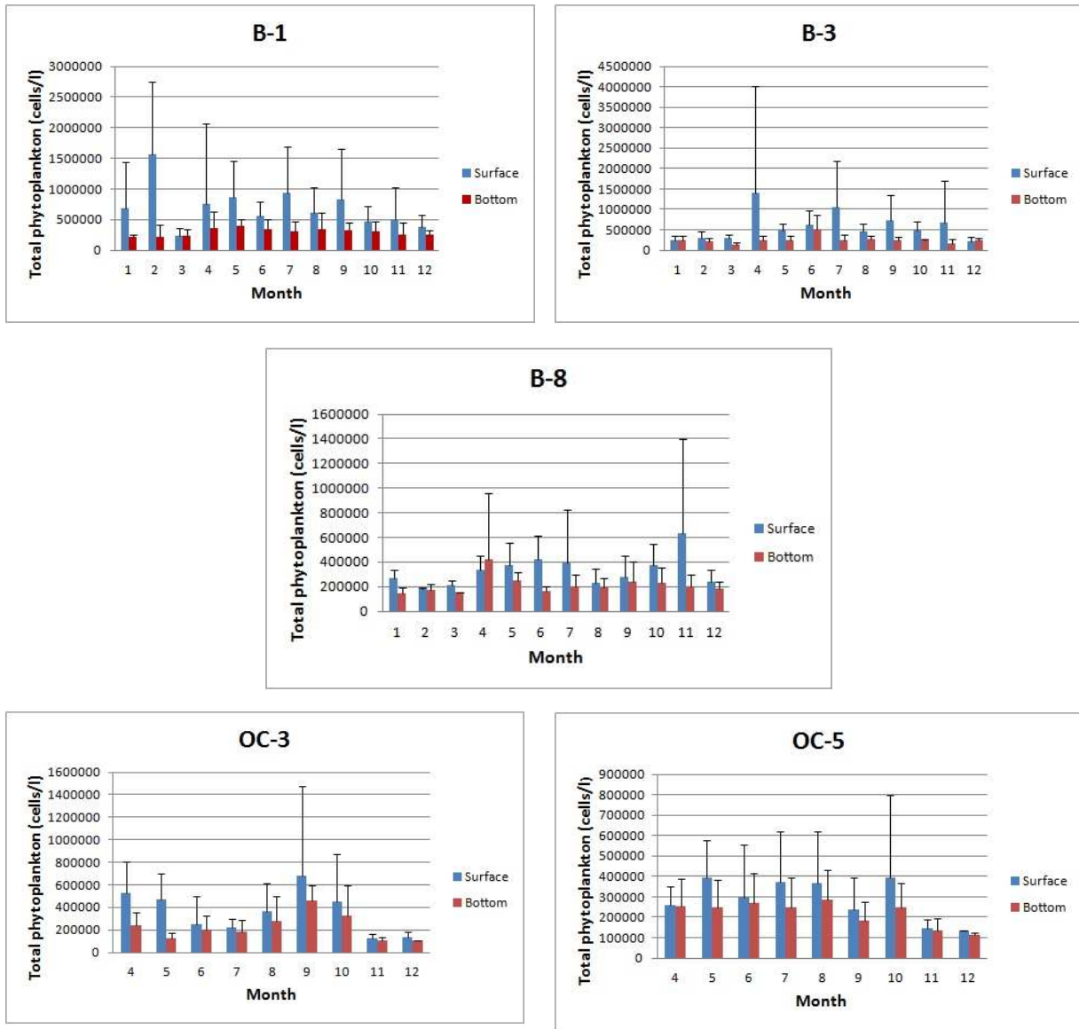
Slika 2.22: Srednje mjesečne vrijednosti (barovi) brojnosti totalnog fitoplanktona sa standardnim devijacijama (vertikalne crte) u površinskom i pridnenom sloju na lokalitetima u zalivskom (B-1, B-3 i B-8) i priobalnom dijelu otvorenog mora (OC-3 i OC-5) u periodu 2009-2019. godine.
