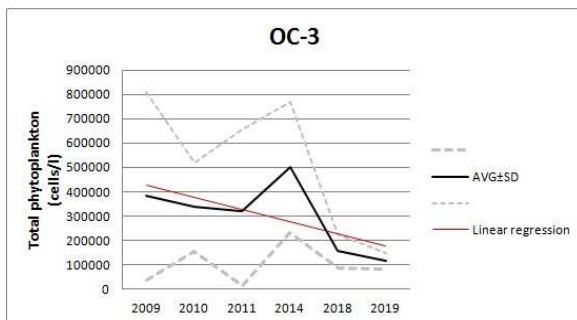
Slika 2.23: Srednje godišnje vrijednosti i standardne devijacije brojnosti fitoplanktona na lokalitetima u zalivskom (B-1, B-3, B-8) i u priobalnom dijelu otvorenog mora (OC-3 i OC-5) Crnogorskog primorja u periodu istraživanja 2009-2019. godine
