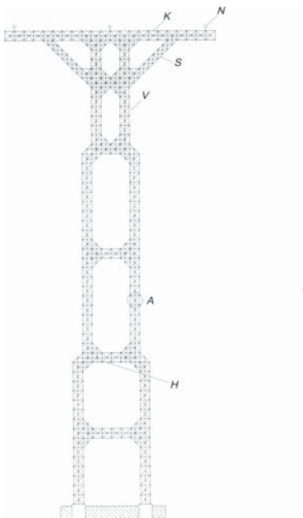
Slika 1. Stub od čelika ili Al-legure „BUMING“- Tip I
