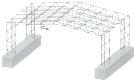
Slika 1. LAKA NOSEĆA PROSTORNA KONSTRUKCIJA HALE SA DVA NAGIBA KROVA "HAMING"
