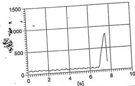
Zadnja osovina
