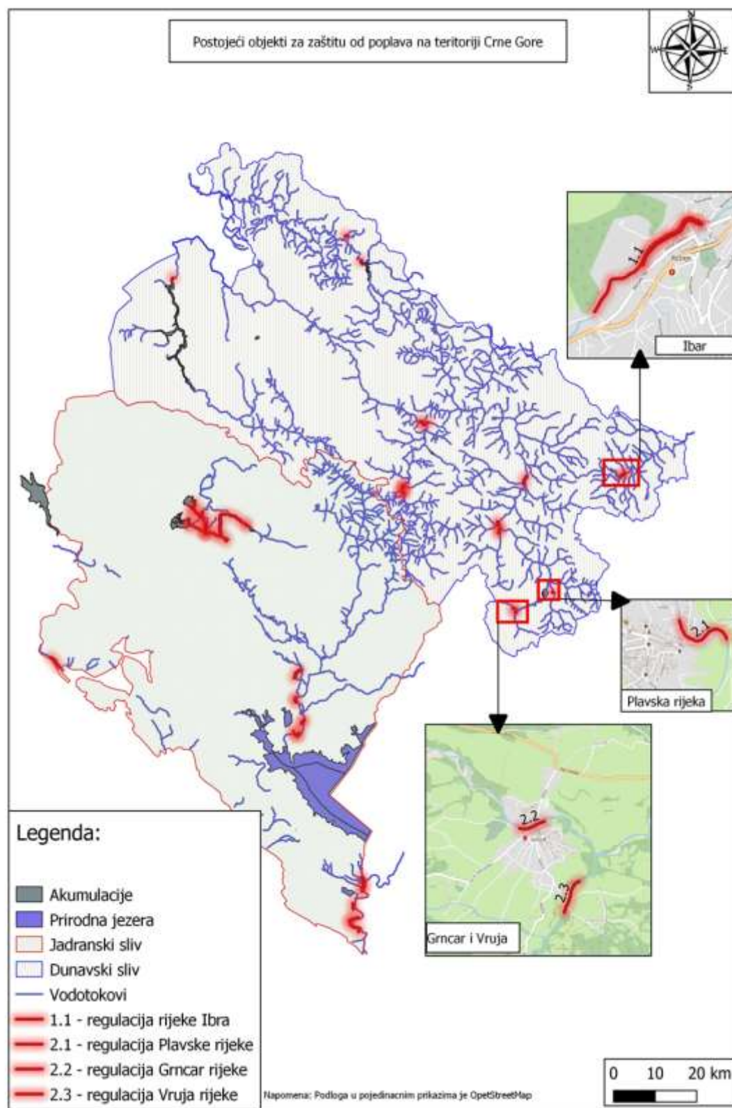
Slika 4.3. Postojeći objekti za zaštitu od poplava na Ibru, Plavskoj rijeci, Grnčaru i Vruji
