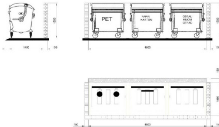
Dimenzije kontejnerskog boksa za 3 kontejnera kapaciteta 1,1\text{m}^3
