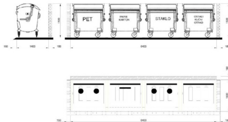
Dimenzije kontejnerskog boksa za 4 kontejnera kapaciteta 1,1\text{m}^3
