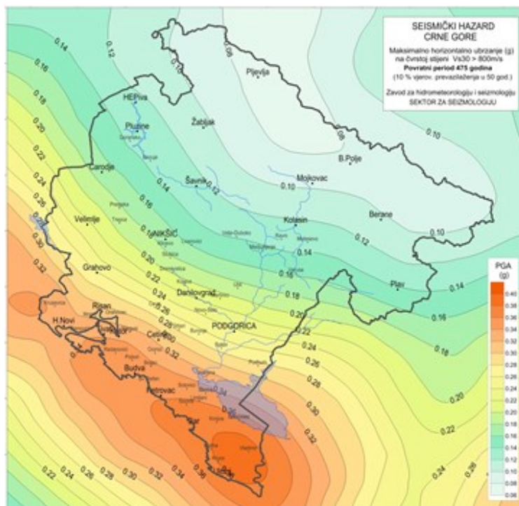
Slika 6: Seizmički hazard za Izmjene i dopune DSL "Dio Sektora 22 i Sektor 23": Očekivano max horizontalno ubrzanje izraženo u djelovima g- za povratne periode od 475 godina izračunato za tlo koje prema Eurokodu 8 kategorisano klasom A (Zavod za hidrometeorologiju i seizmologiju, 2015).
