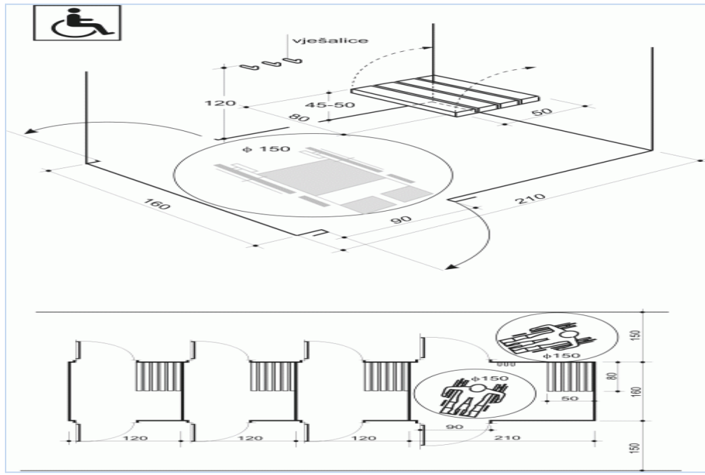
Grafički prikaz br. 25 - Kabina za presvlačenje – iz člana 25 Pravilnika
