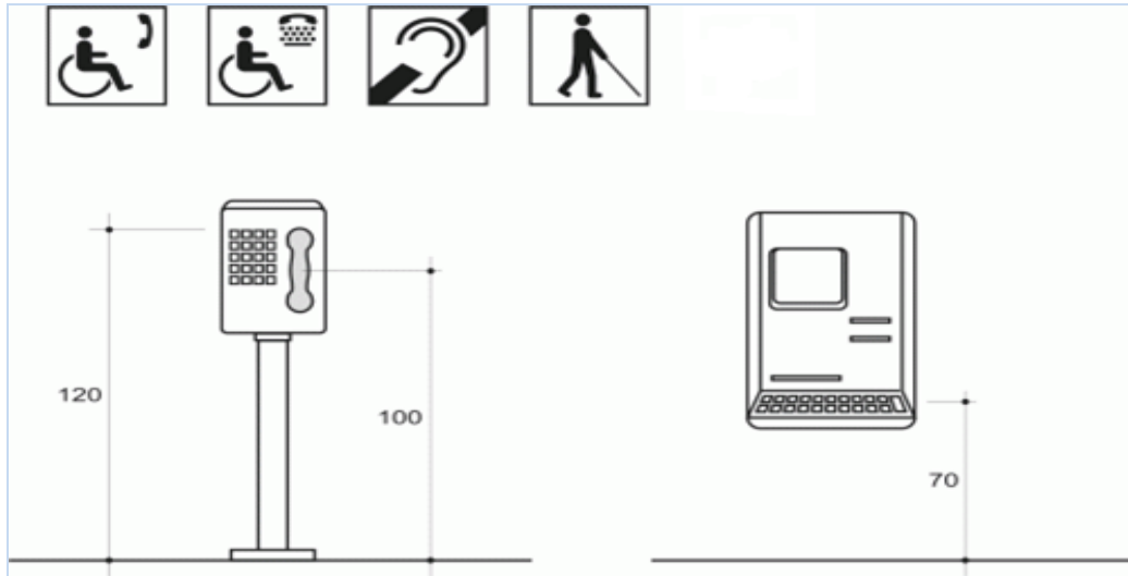
Grafički prikaz br. 31 - Telefon, tekstofon, faks, bankomat – iz člana 30 Pravilnika
