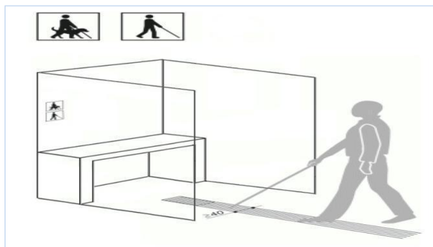
Grafički prikaz br. 28 - Glasачka kabina za lica sa oštećenjem vida – iz člana 27 Pravilnika
