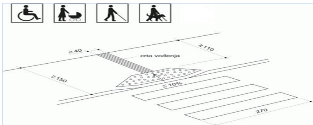
Grafički prikaz br. 40 - Pješački prelaz izvan ukrštanja – iz člana 43 stava 1 alineje 4 Pravilnika
