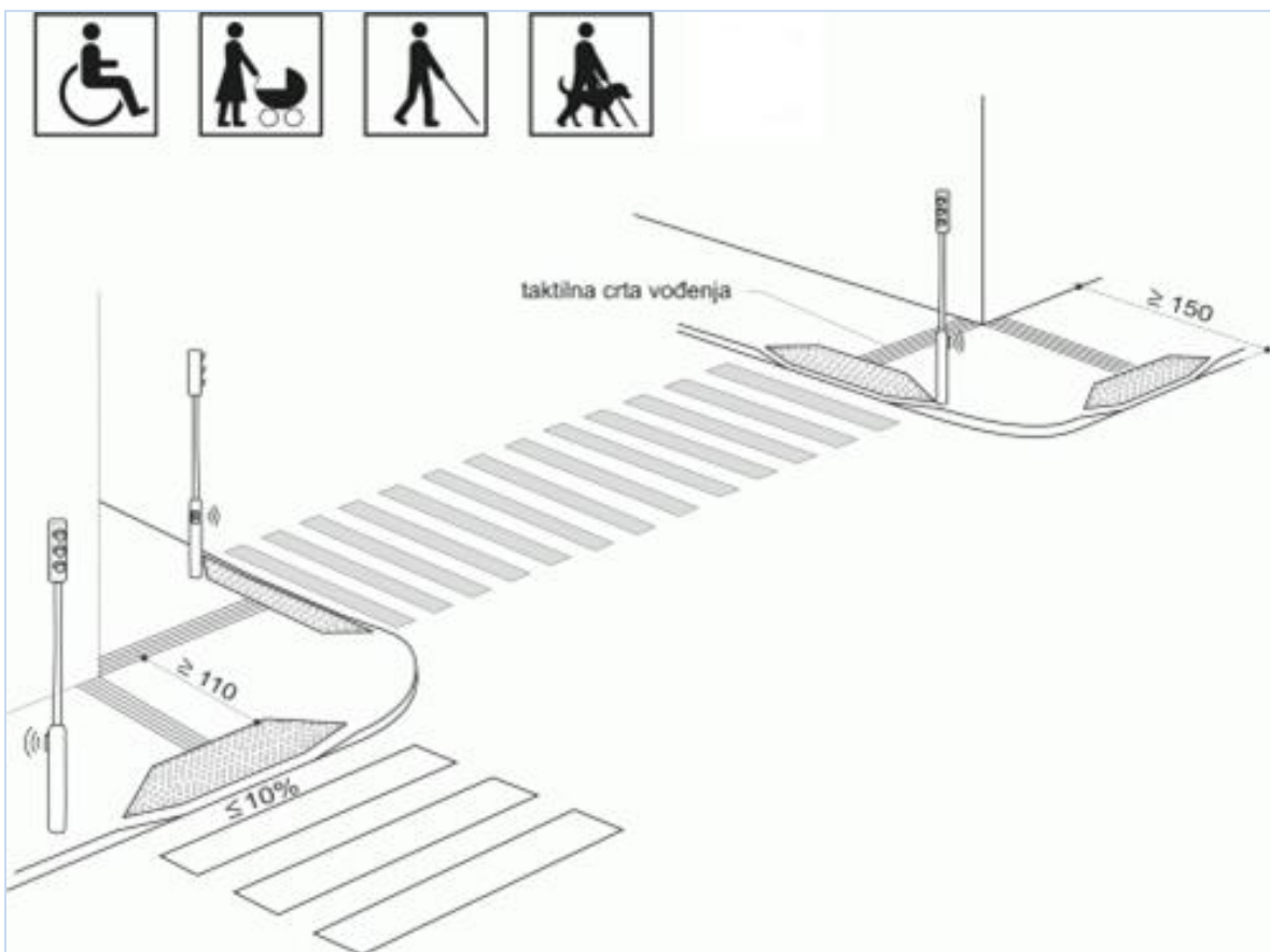
Grafički prikaz br. 42 - Rakrsnica – iz člana 45 Pravilnika
