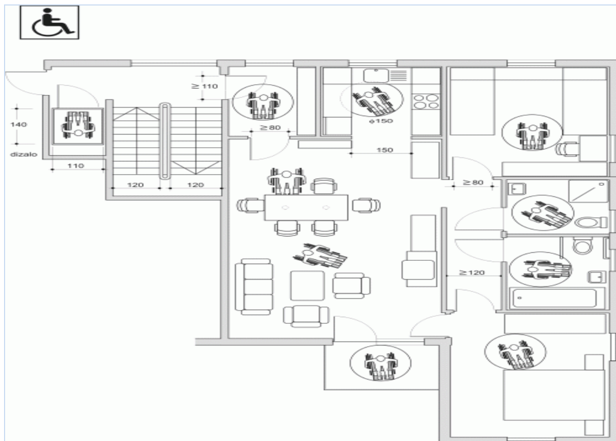
Grafički prikaz br. 22 - Stan – iz člana 23 Pravilnika
