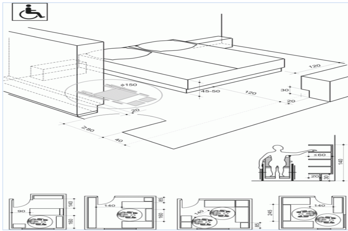
Grafički prikaz br. 19 - Soba – iz člana 22 Pravilnika
