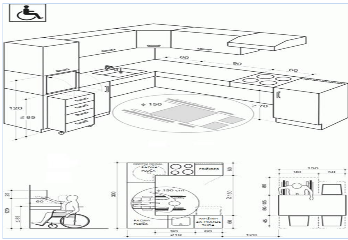
Grafički prikaz br. 18 - Kuhinja – iz člana 21 Pravilnika
