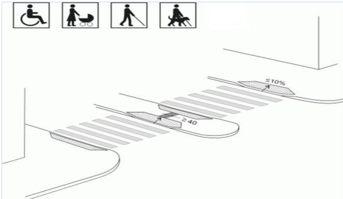
Grafički prikaz br. 41 - Pješačko ostrvo – iz člana 44 stava 1 alineje 3 Pravilnika
