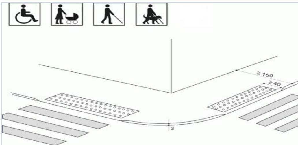
Grafički prikaz br. 40 - Pješački prelaz izvan ukrštanja – iz člana 43 stava 1 alineje 4 Pravilnika
