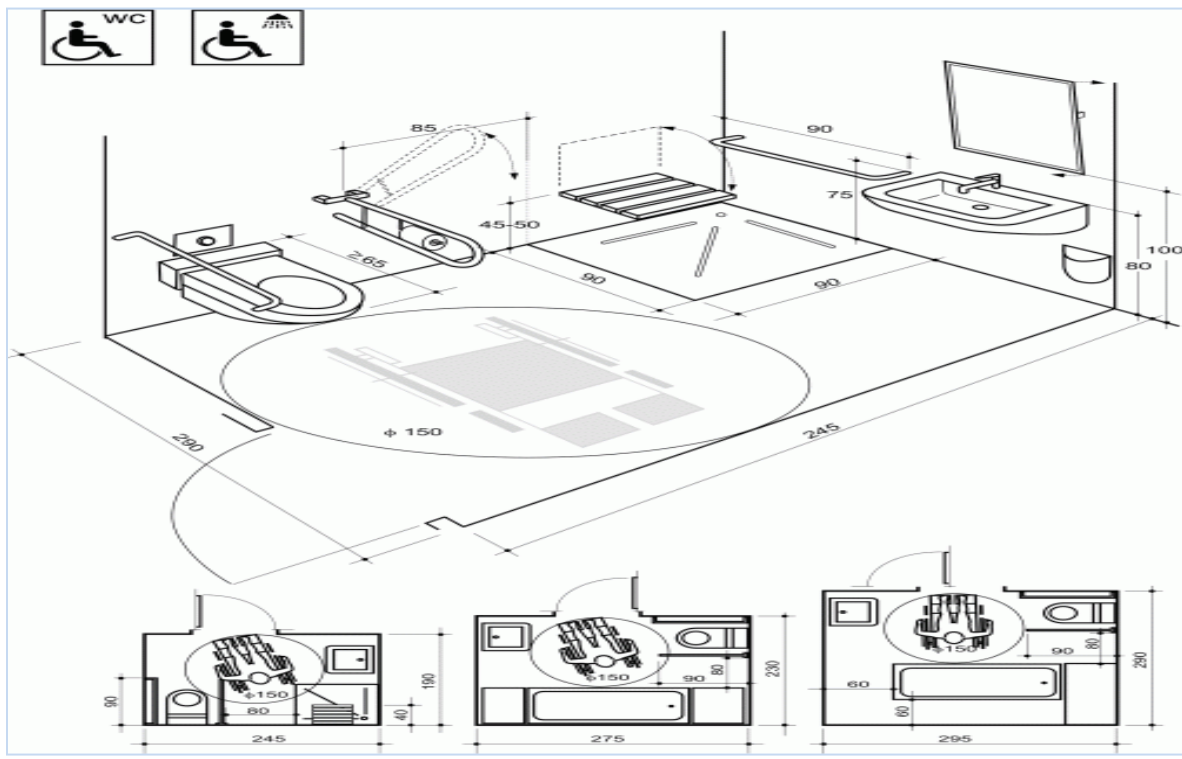
Grafički prikaz br. 17 - Kupatilo – iz člana 20 Pravilnika
