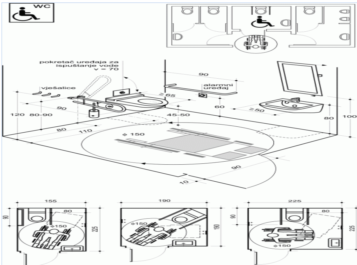
Grafički prikaz br. 16 - WC – iz člana 19 Pravilnika
