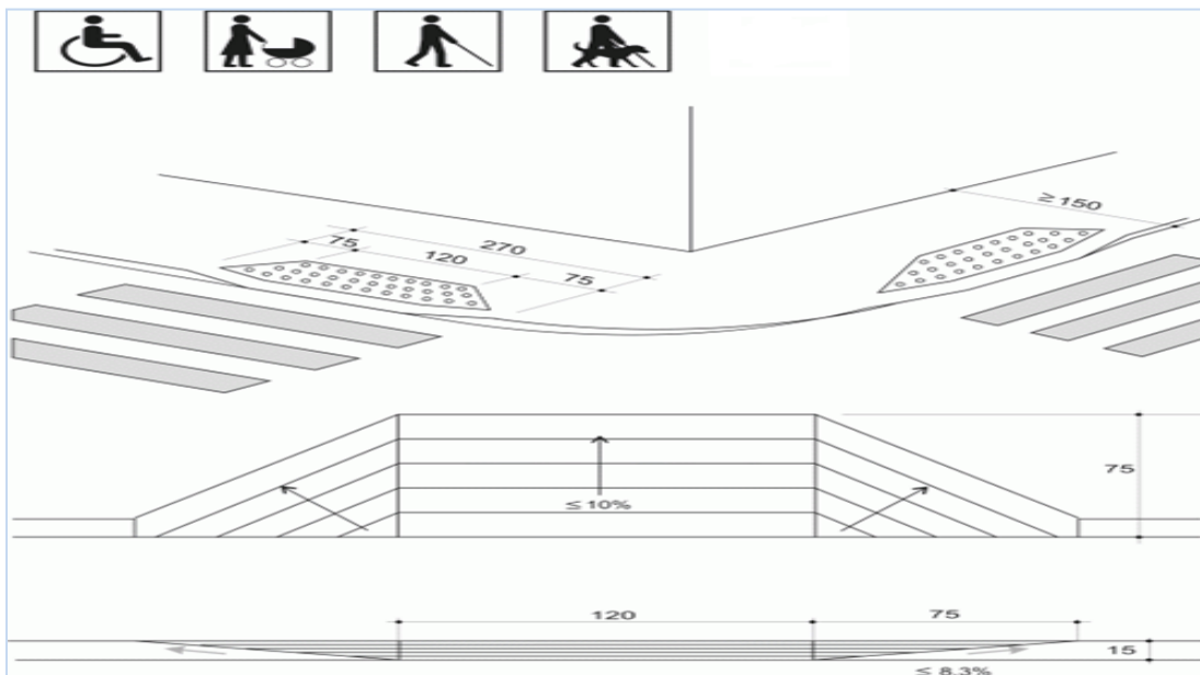
Grafički prikaz br. 39 - Pješački prelaz na mjestu najmanje visine trotoara – iz člana 43 stav 1 alineja 3 Pravilnika
