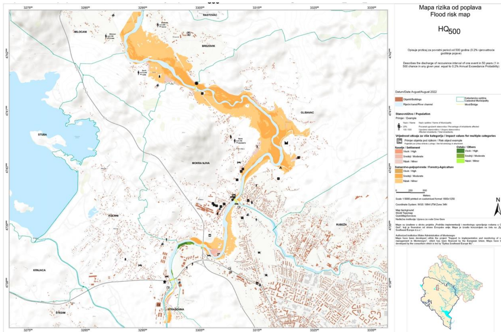
Slika 6.4. Obim poplave za APSFR20_ARB_Zeta01 (južni region)
