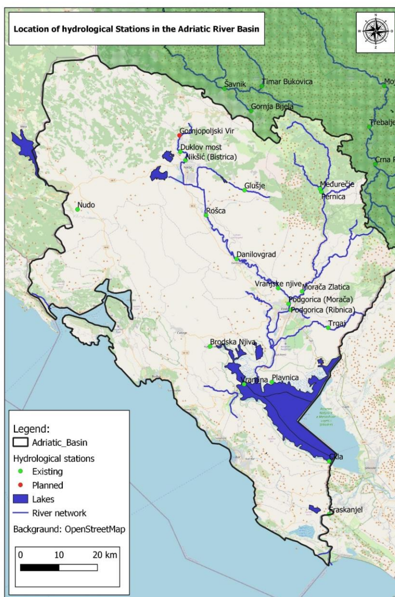
Slika 4.1. Hidrološke stanice na vodnom području Jadranskog sliva
