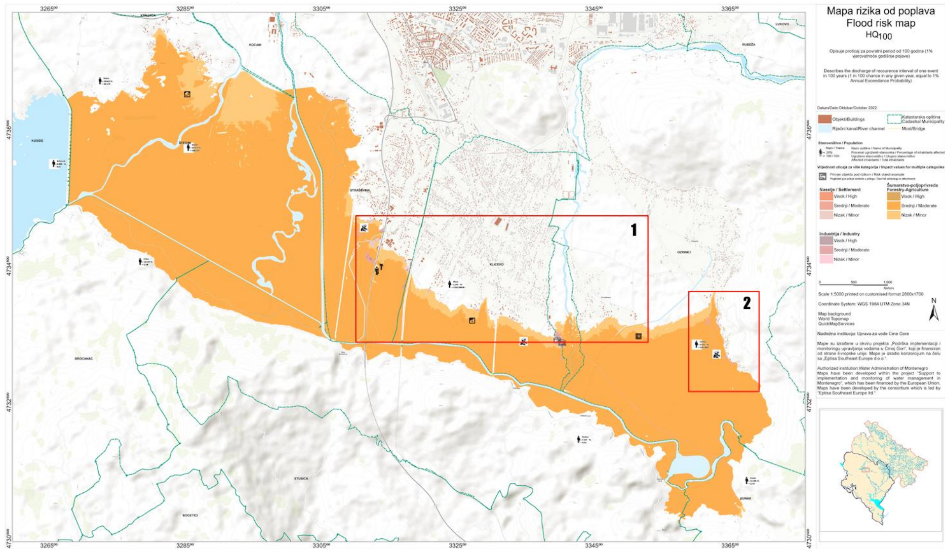
Slika 8.2. Identifikovane oblasti potencijalnih poplava u APSFR20_ARB_Zeta01 južni region (HQ100)
