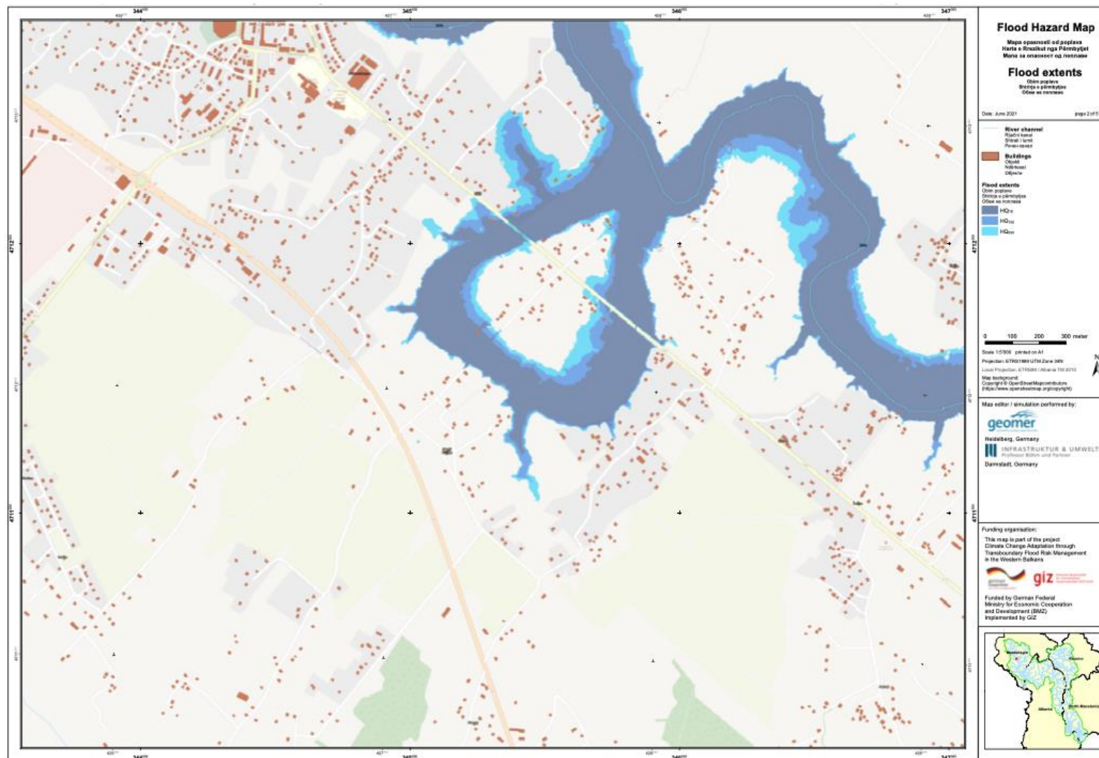
Slika 6.11. Obim poplave za APSFR21_ARB_Zeta02 (Sekcija 2)
