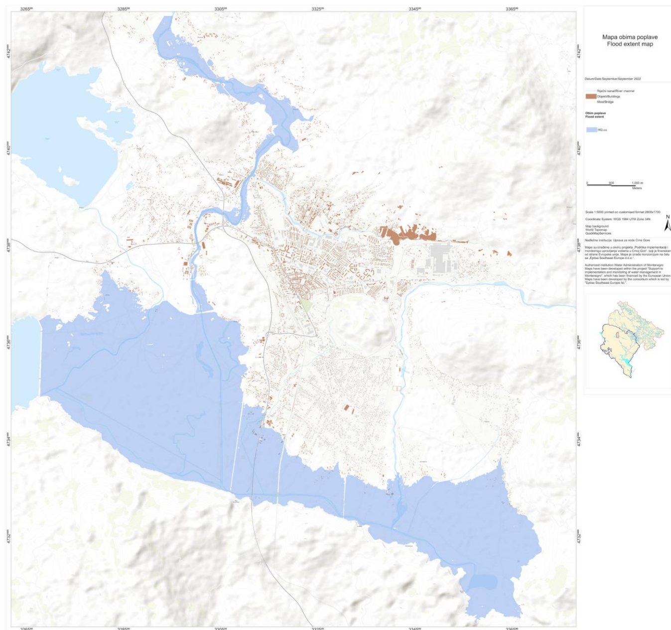
Slika A4.1 Obim poplava u APSFR20_ARB_Zeta01 (HQ100) – sjeverni i južni regioni zajedno
