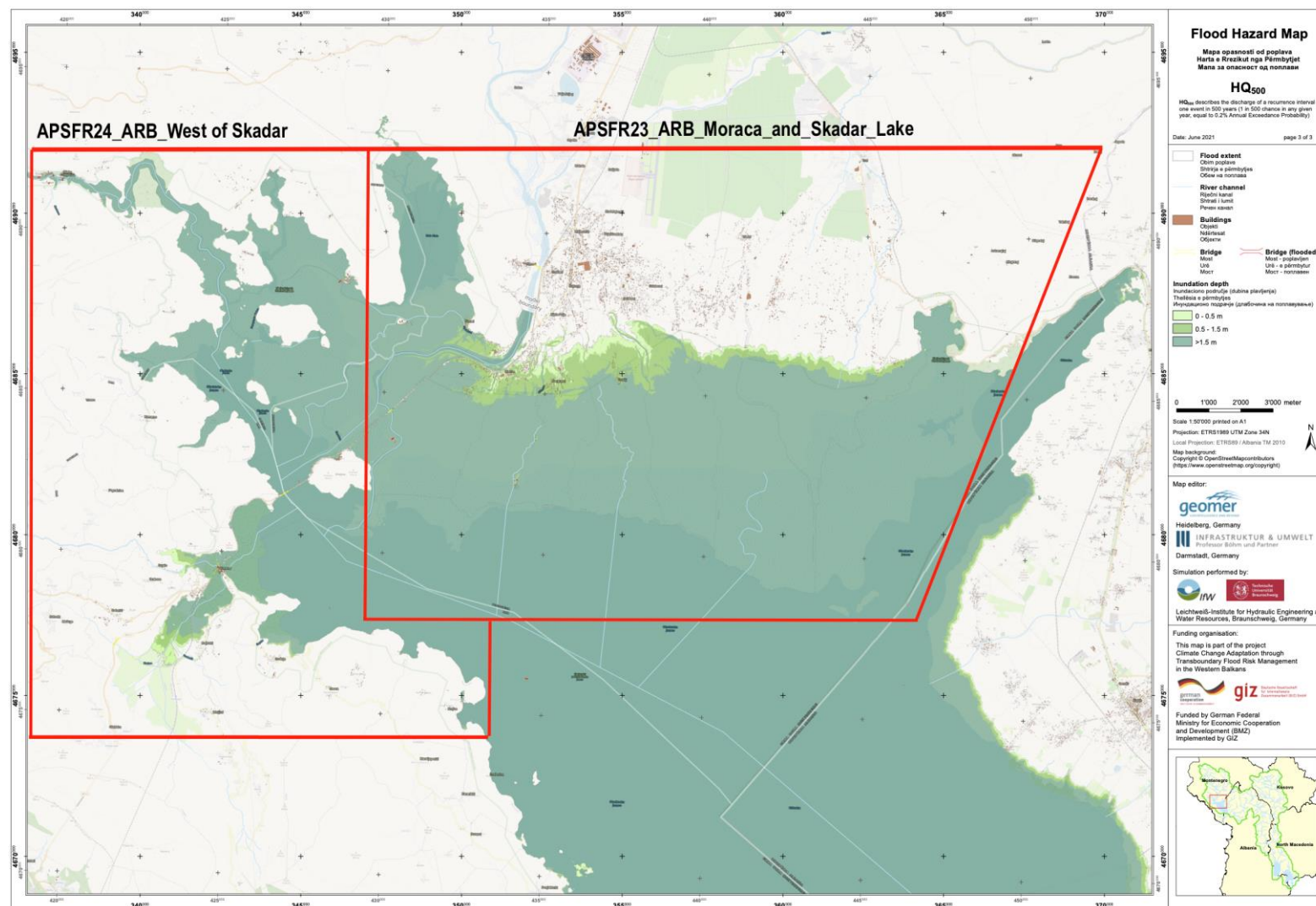
Slika 6.27. Dubina plavljenja (HQ500) za APSFR23_ARB_Morača i Skadarsko jezero01 i APSFR24_ARB_Skadarsko jezero02
