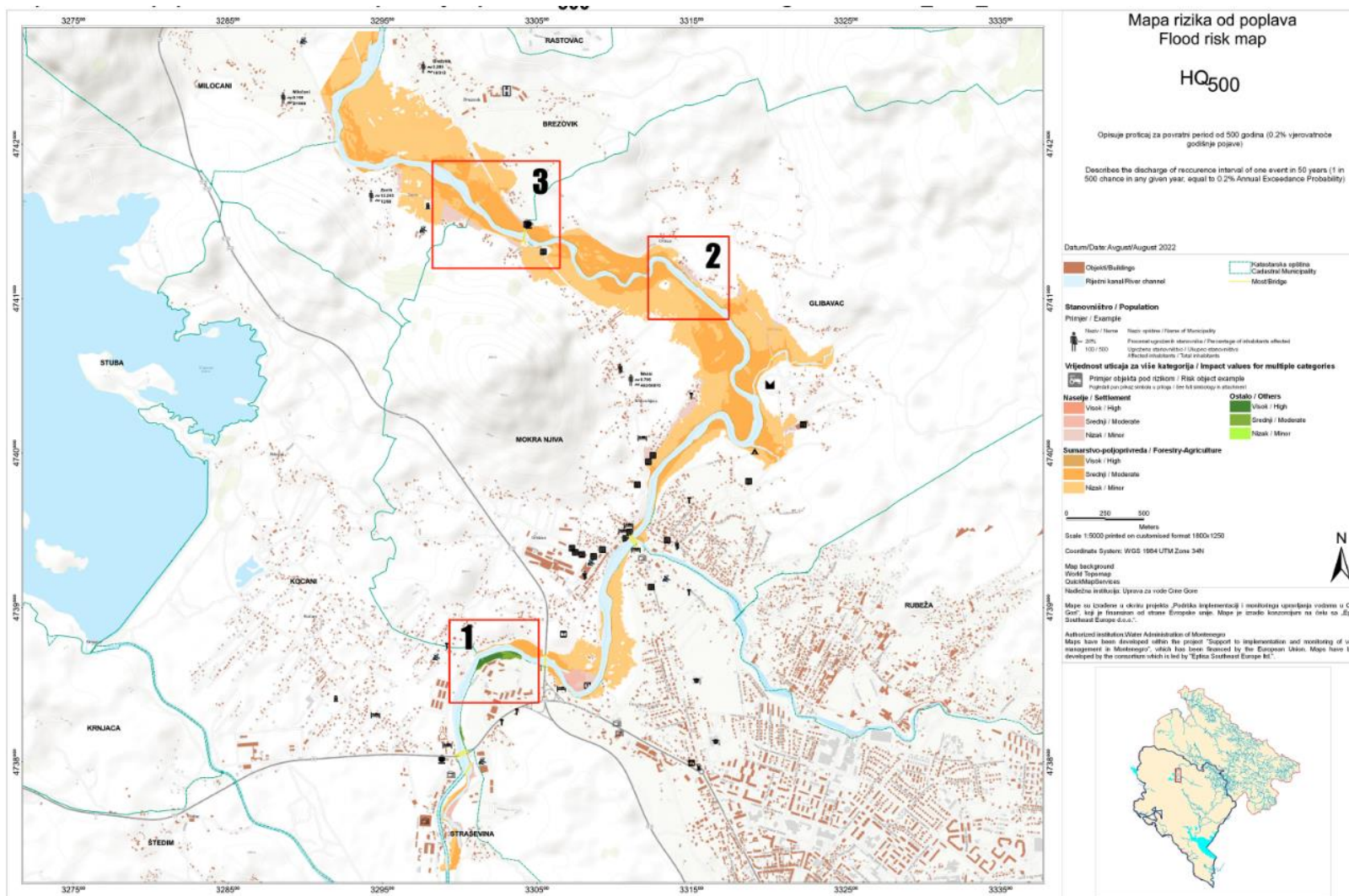
Slika 8.1. Identifikovane oblasti potencijalnih poplava u APSFR20_ARB_Zeta01 sjeverni region (HQ500)
