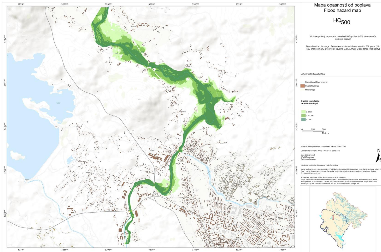
Slika 6.2. Dubina plavljenja (HQ500) za APSFR20_ARB_Zeta01 (Sjeverni region)
