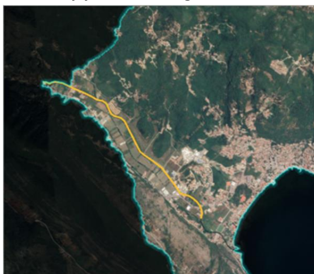
Slika 4.3. Dionica Sutorine na kojoj su izvođeni regulacioni radovi
