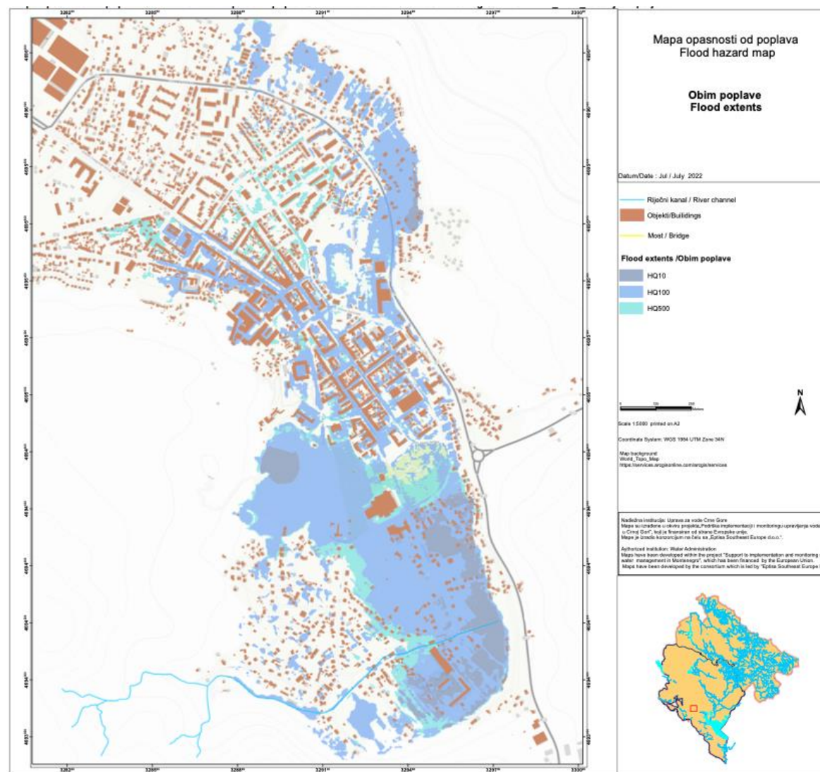
Slika 6.23. Obim poplave za APSFR22_ARB_ podzemne vode Cetinjskog polja01
