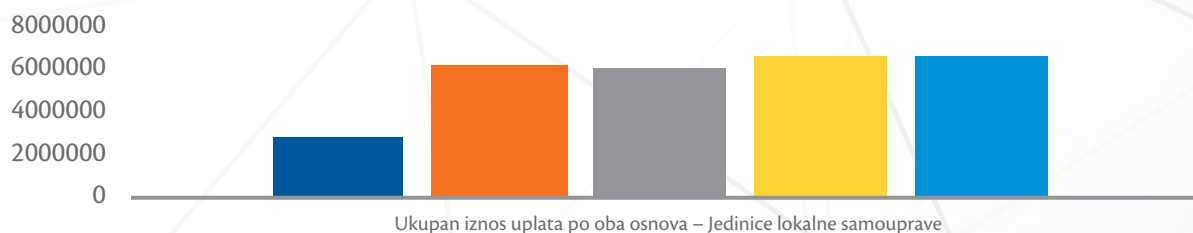
Grafikon 6: Poređenje ukupnih podataka dostavljenih od strane jedinica lokalne samouprave shodno izvještajnim godinama
