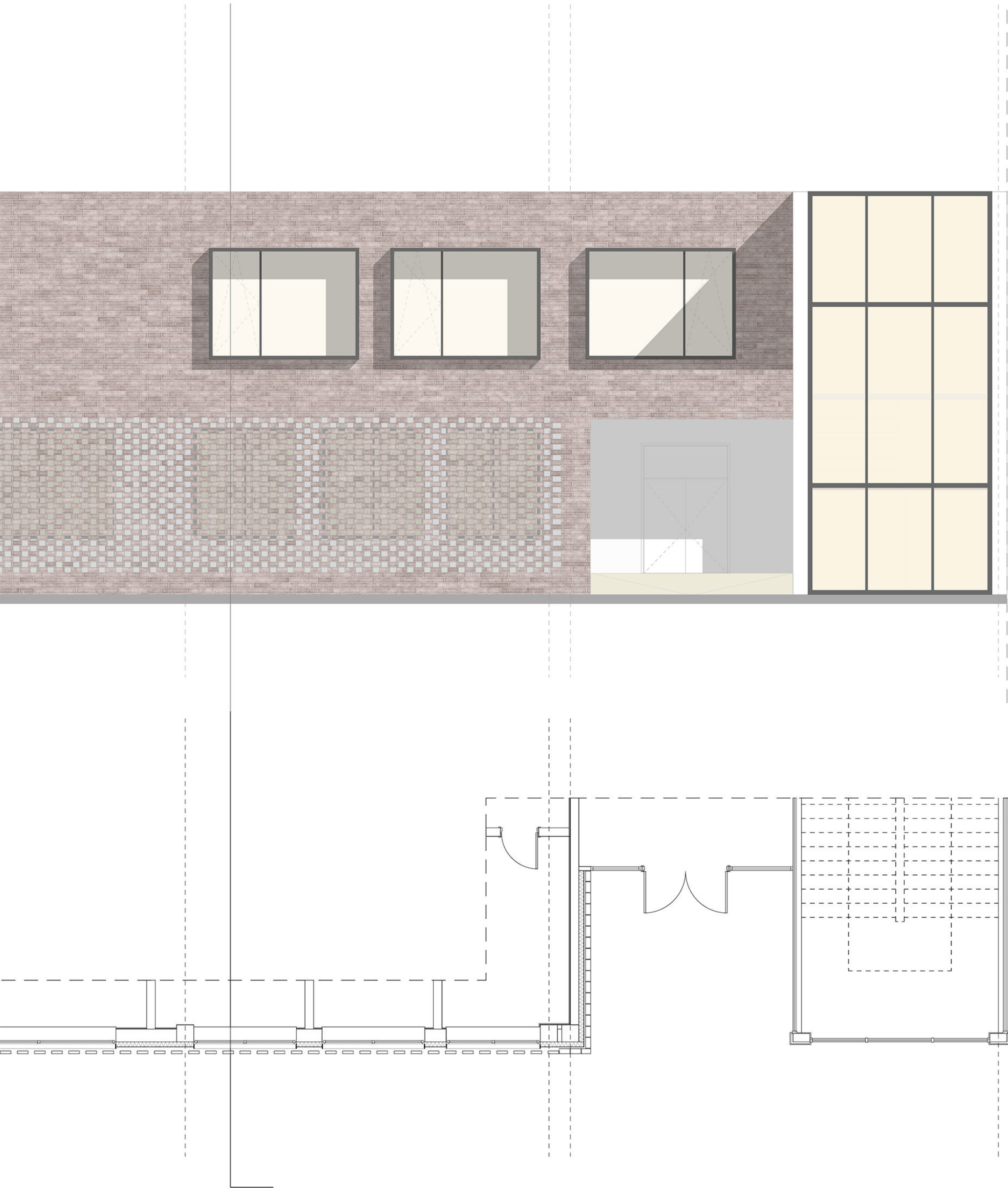
DETALJ FASDE 1:50
