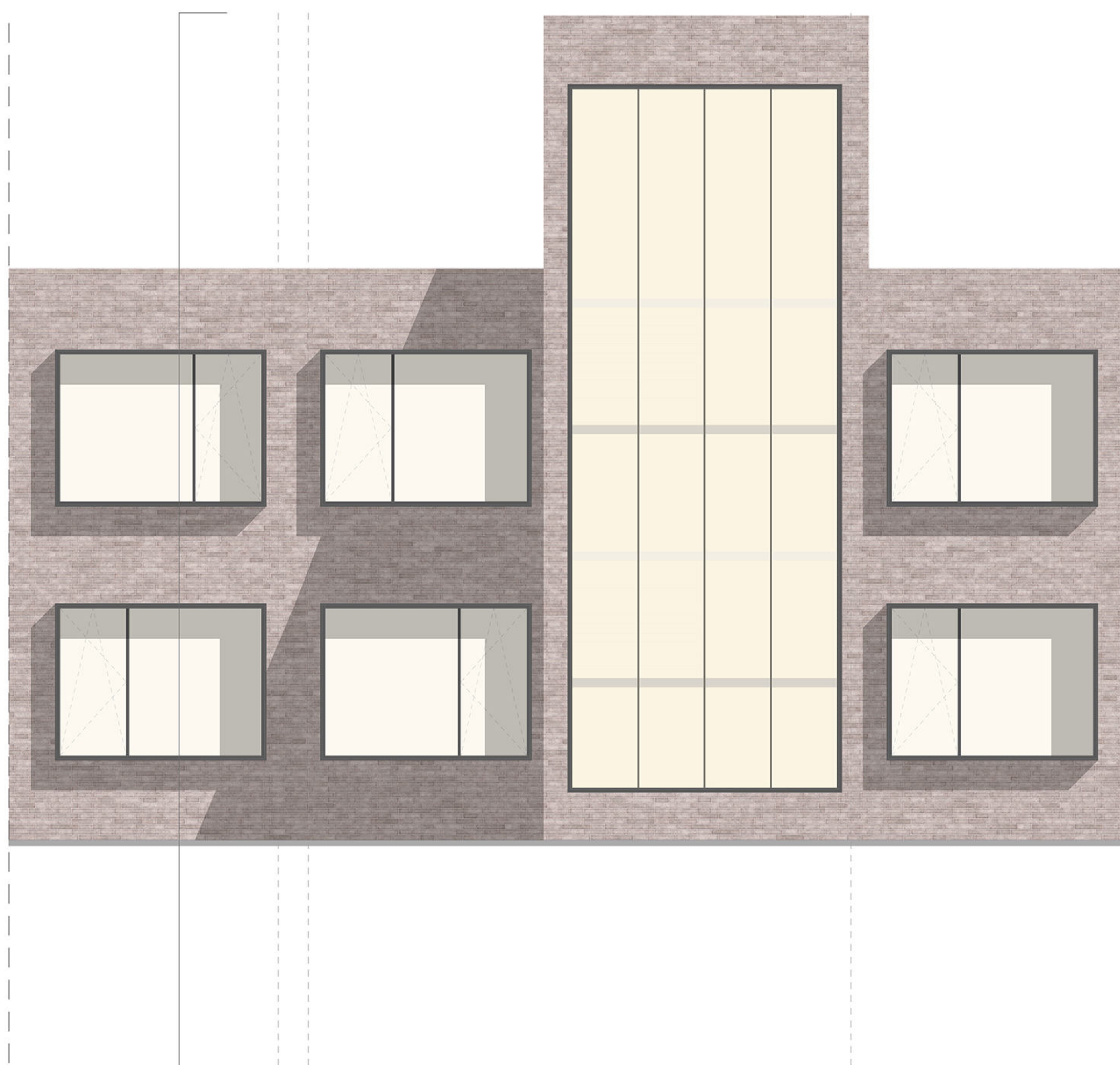
DETALJ VENTILIRANE FASADE 1:50
