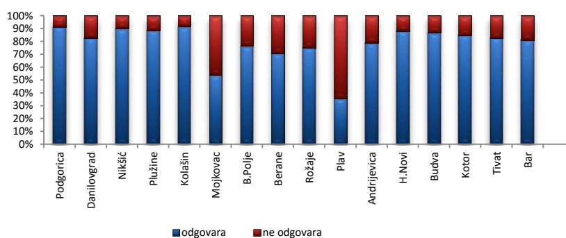
Grafikon 49. Rezultati fizičko-hemijskih ispitivanja uzoraka hlorisane vode za piće
