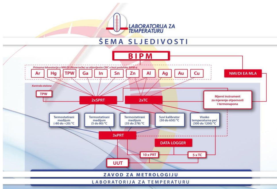
Slika 7. Lanac sljedivosti u oblasti mjerenja temperaturu
