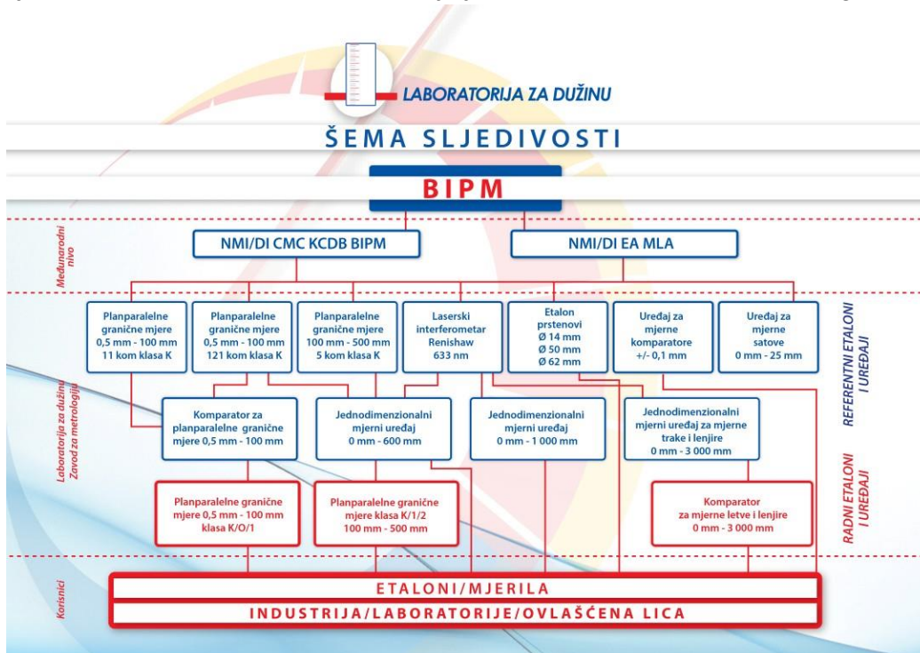
Slika 6. Lanac sljedivosti u oblasti mjerenja dužine
