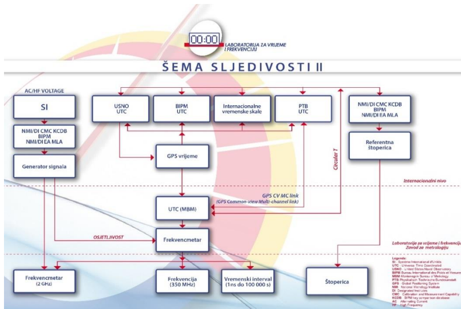
Slika 10. Lanac sljedivosti oblasti mjerenja vremena i frekvencije
