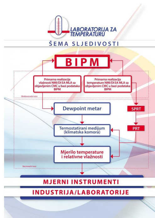
Slika 8. Lanac sljedivosti u oblasti mjerenja relativne vlažnosti
