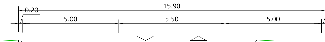
PRESJEK 12-12 (Ulica 12)
