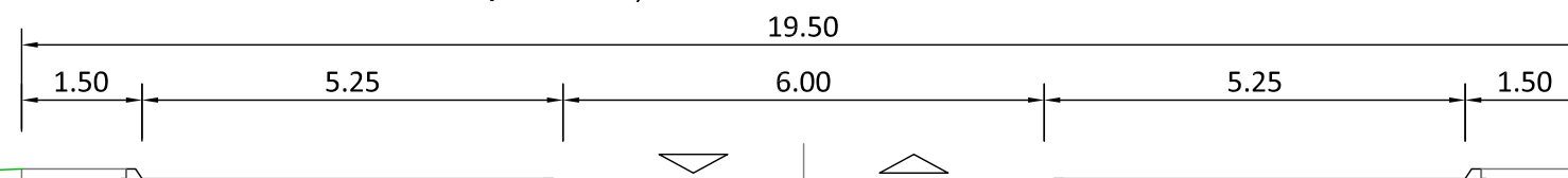
PRESJEK 10-10 (Ulica 9)
