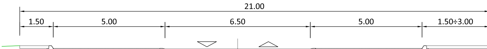
PRESJEK 2-2 (Ulica 1, Ulica 4, Ulica 7)
