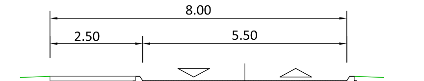
PRESJEK 14-14 (Ulica 3')
