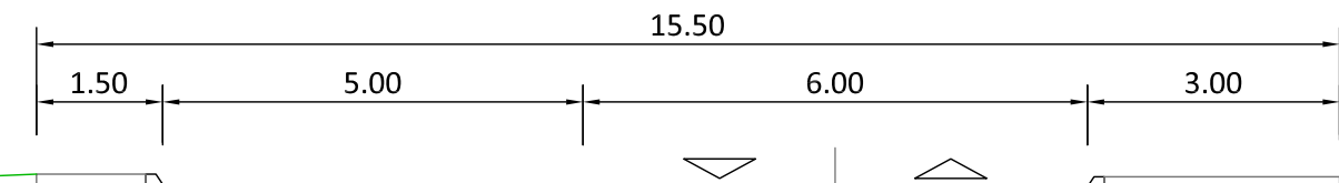
PRESJEK 8-8 (Ulica 6)
