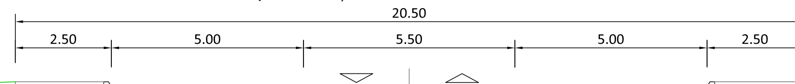
PRESJEK 11-11 (Ulica 11)
