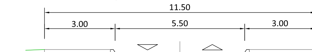
PRESJEK 6-6 (Ulica 3)
