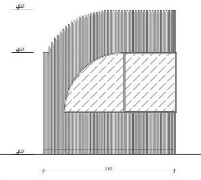
pogled 4, R 1:50
