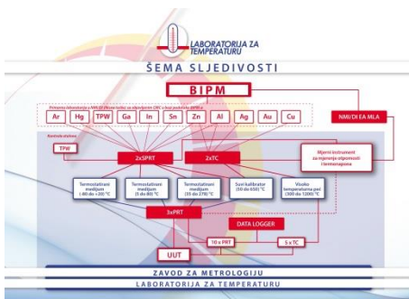
Šema sljedivosti Laboratorije za temperaturu
