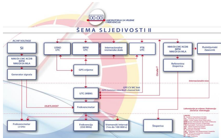
Šema sljedivosti Laboratorija za vrijeme i frekvenciju
