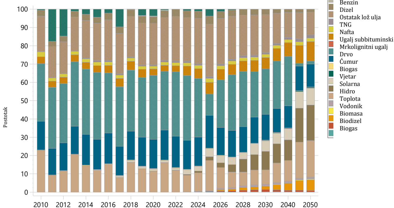
Slika 5.7 Udio snabdijevanja primarnom energijom po gorivima (u %) za istorijske godine 2010-2022, i predviđanja do 2050. godine uz dodatne mjere
