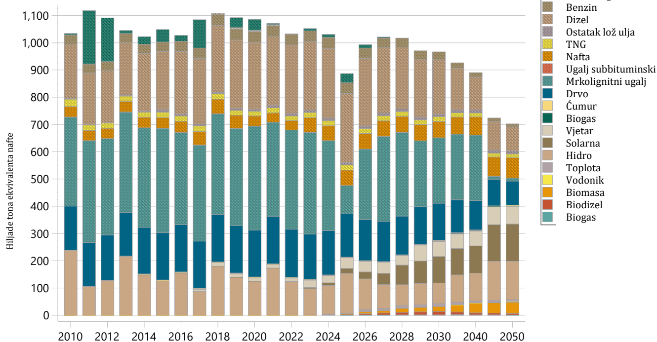
Slika 5.6 Snabdijevanje primarnom energijom po gorivima (u ktOE) za istorijske godine 2010-2022, i predviđanja do 2050. godine uz dodatne mjere
