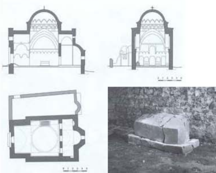
Osnova crkve na Zagrađu, ktitora Stefana Vukčića Kosače, (prema M. Kovačeviću) i Stećak ktitora uz sjeverni zid crkve na Zagrađu, poslije istraživanja i anastiloze 1973. godine
