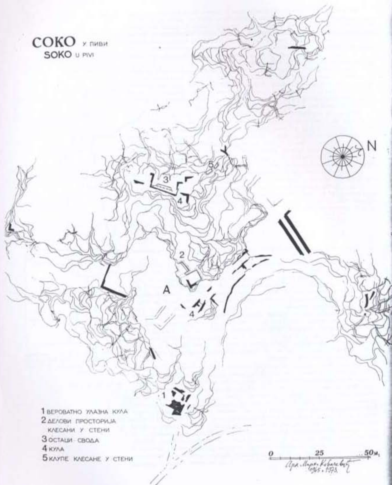
СА. 110 Соко у Пиви, план града — Fig. 110 Soko u Piva, plan
