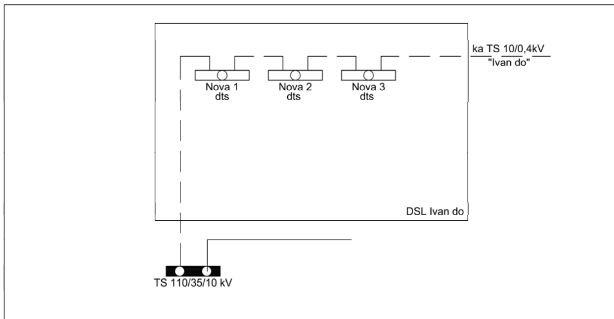
Slika. Jednopolna šema 10 kV mreže, novoplanirano stanje
