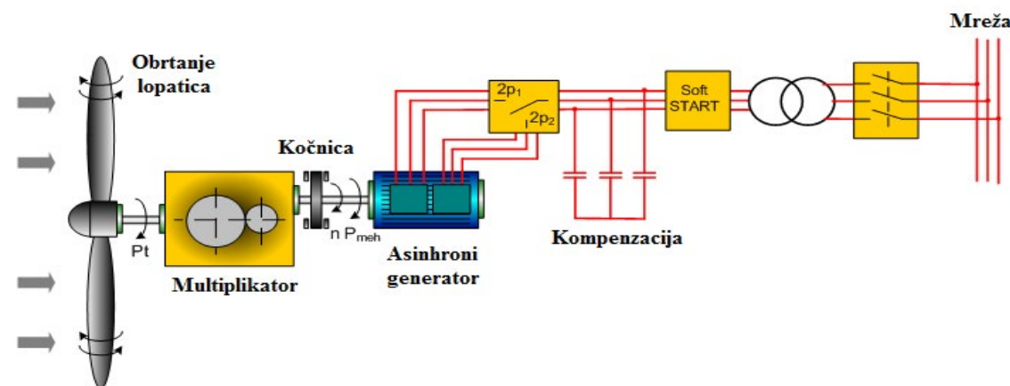
VA sa indukcionim kaveznim vjetrogeneratorom
