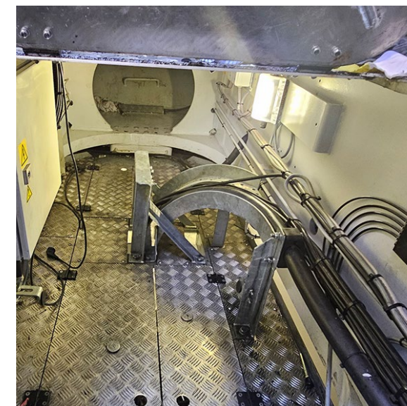
Polaganje i povezivanje napojnih kablova unutar gondole vjetroturbine
