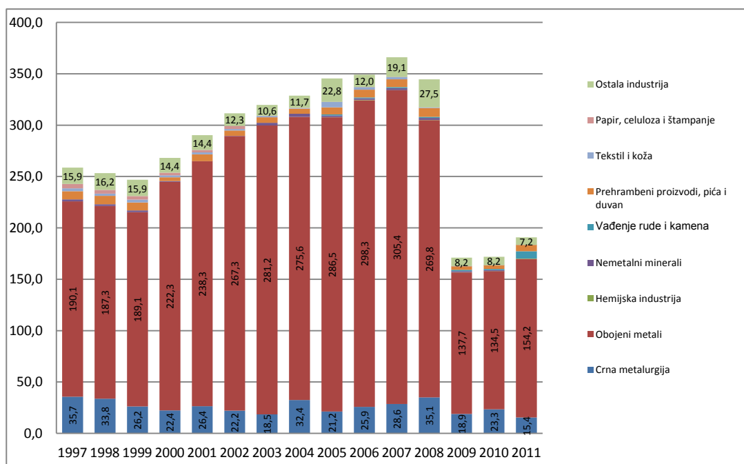
Slika 7: Potrošnja finalne energije po industrijskim granama, 1997-2011 (ktce)
