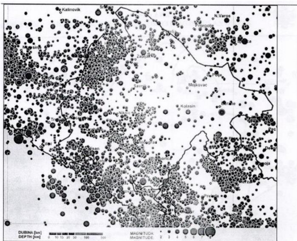
Slika 1. Karta svih epicentara zemljotresa 1444-2022, M>2
