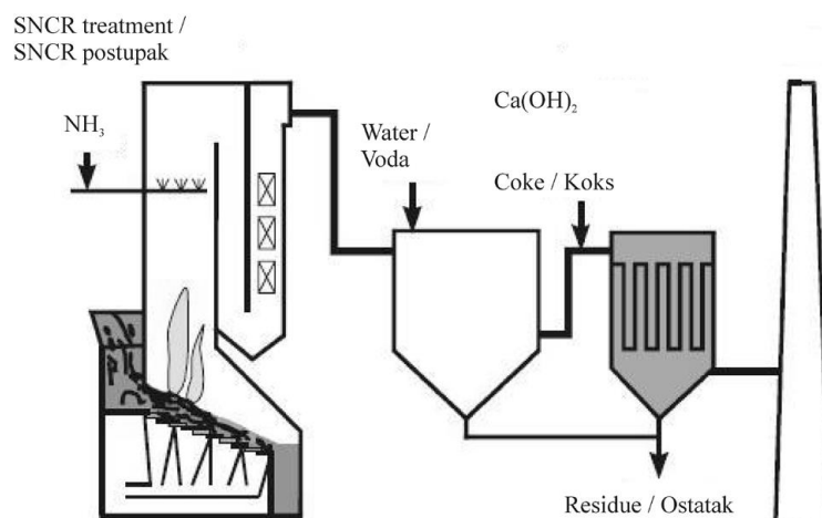
Slika 41. Šematski prikaz prečišćavanja dimnih gasova – varijanta 1
