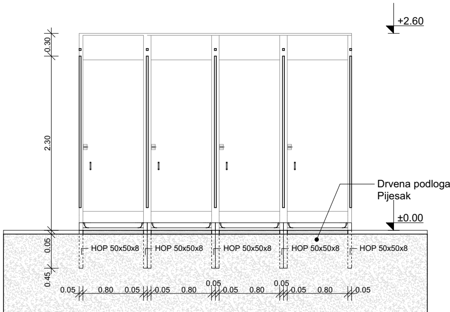
PRESJEK 1-1
