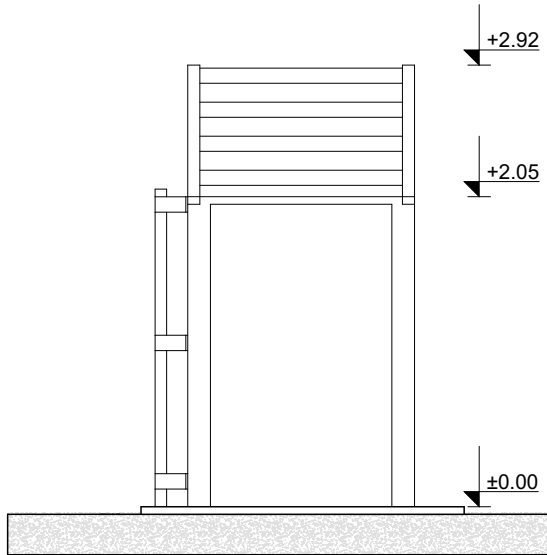
IZGLED 2
