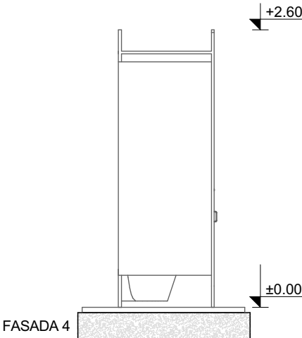
FASADA 4
