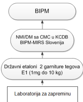
Slika 8. Lanac sljedivosti u oblasti zapremine
