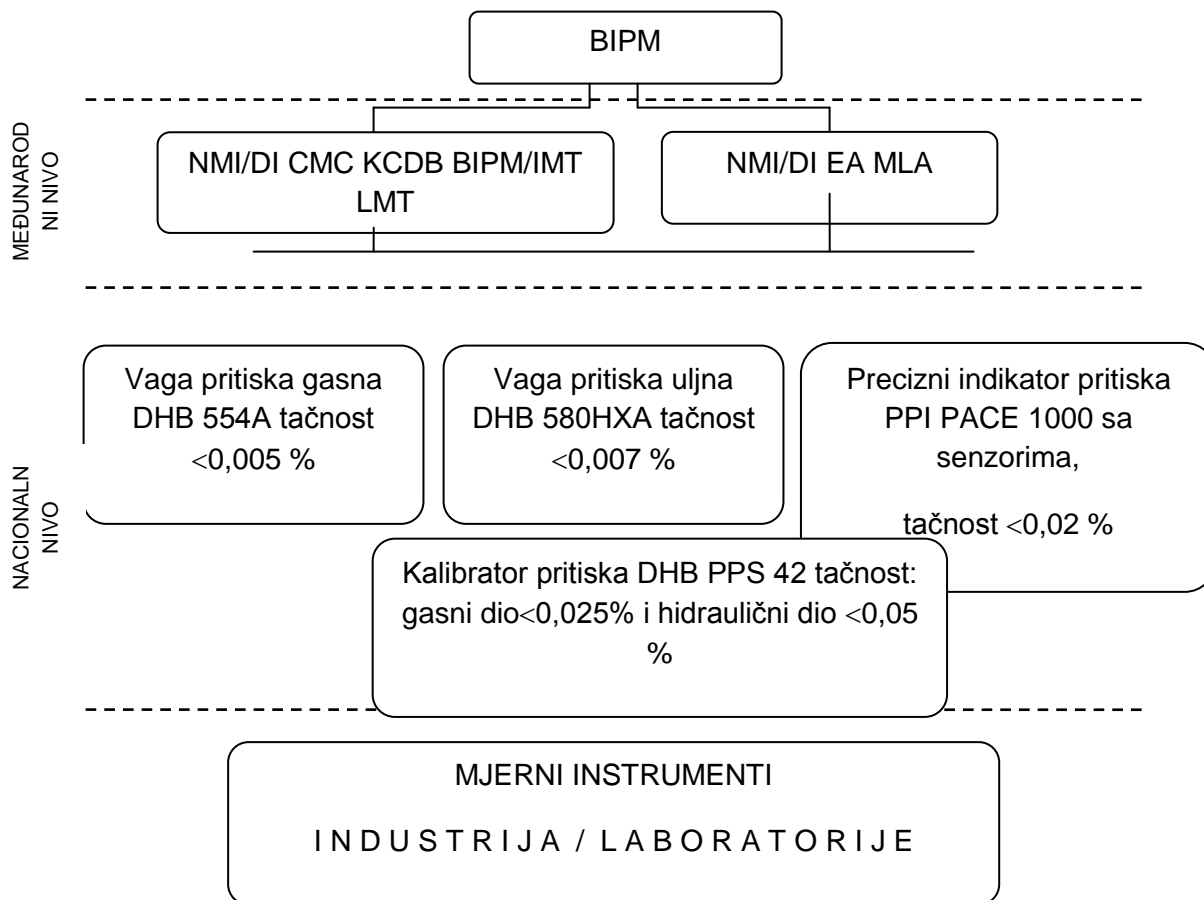
Slika 4. Lanac sljedivosti u oblasti mjerenja pritiska
