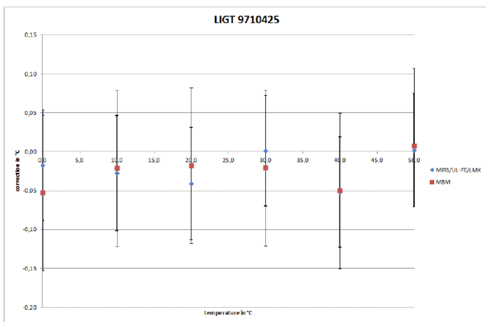
Slika 8. Rezultati poređenja kalibracija živinog termometra (opseg od 0°C do 50°C)
