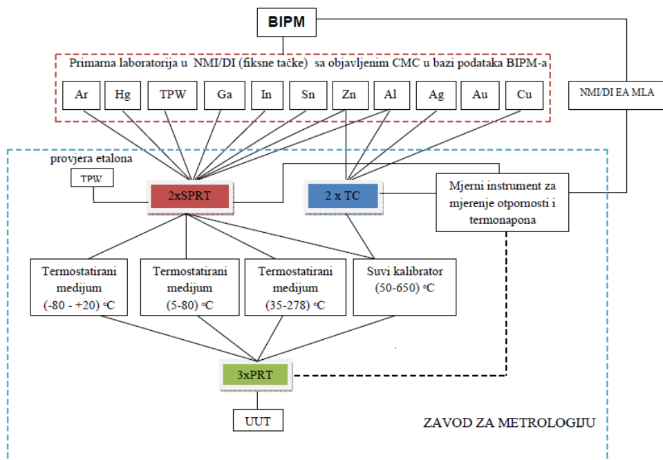
Slika 3. Lanac sljedivosti u oblasti mjerenja temperature
