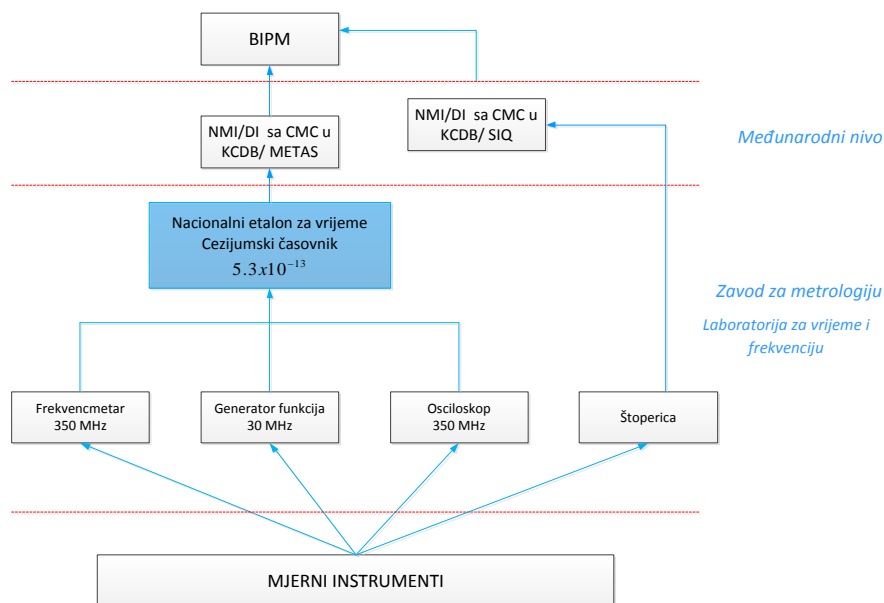
Slika 7. Lanac sljedivosti u Laboratoriji za vrijeme i frekvenciju
