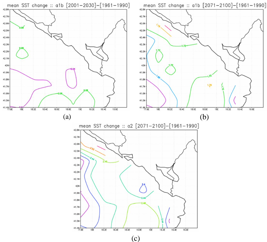
Slika 6.14: Promjene srednje godišnje temperature mora u °C za primorje Crne Gore, (a) za period 2001-2030. i scenario A1B, (b) za period 2071-2100. i scenario A1B, (c) za period 2071-2100. i scenario A2.
