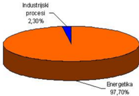
Sl. 4.4.: NO x emisija iz ekonomskih sektora (10.35 Gg, 1990.)
