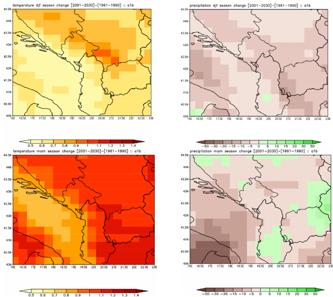
Slika 6.5: Promjene za DJF (gornji paneli) i MAM (donji paneli) sezonu, temperature na 2 m (°C) (paneli lijevo) i akumuliranih padavina (%) (paneli desno) na teritoriji Crne Gore za A1B scenario tokom perioda 2001-2030.
