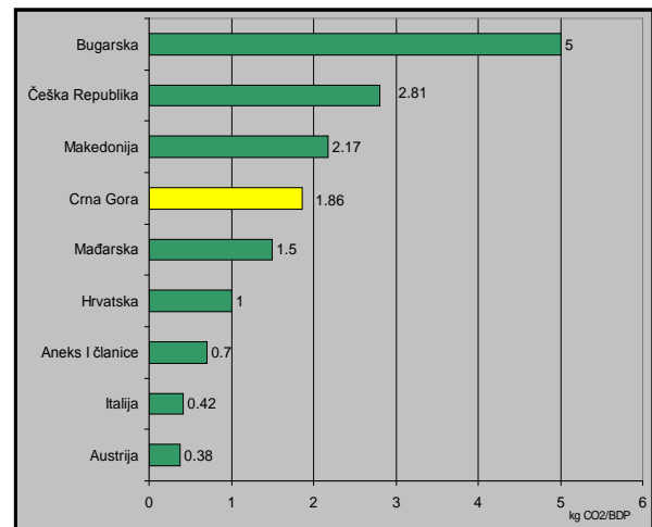
Slika 1.2.: Uporedne CO 2 emisije po kg CO 2 /USD po kursu iz 2000. godine, Crna Gora, zemlje iz regiona, Anex 1 članice (izvor podatak IEA, 2009)
