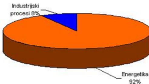
Sl. 4.1.: CO 2 emisija iz ekonomskih sektora (2,691.56 Gg, 1990.)
