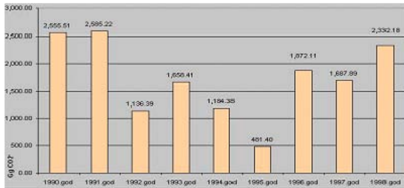
Slika 4.9.: Upporedne CO 2 emisije za period 1990-1998 godina po godinama (referentni pristup).
