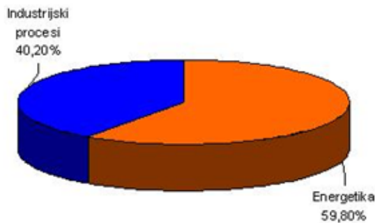
Sl. 4.6.: NMVOC emisija iz ekonomskih sektora (8.92 Gg, 1990.)
