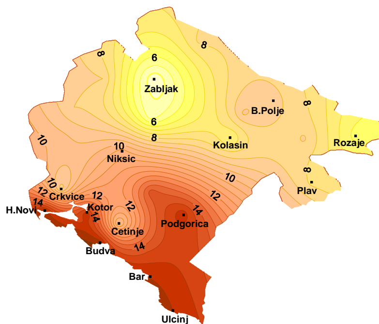
Slika 3.1.: Godišnja raspodjela temperature vazduha (0C) za period osrednjavanja 1961-1990
