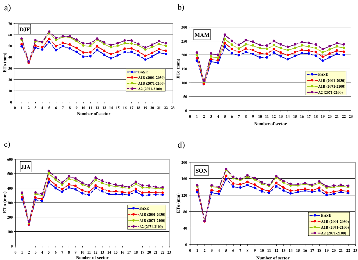
Slika 6.15.: Sumarna referentna evapotranspiracija zimskog perioda DJF (a), prolećnog perioda MAM (b), ljetnjeg perioda JJA (c) i jesenjeg perioda SON (d) za bazni (BASE) i tri buduća klimatska scenarija (A1B (2001-2030), A1B (2071-2100) i A2 (2071-2100))
