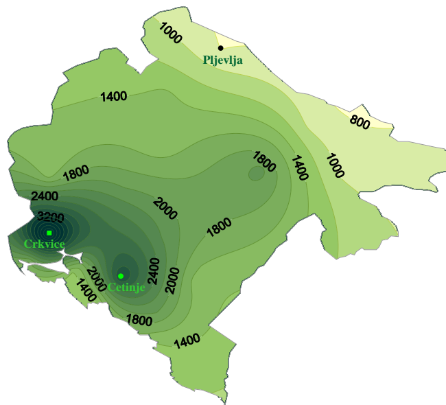
Slika 3.2.: Godišnja raspodjela padavina (mm) za period osrednjavanja 1961-1990
