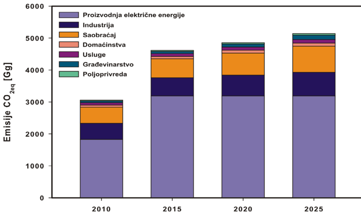
Slika 5.2: Referentni scenario porasta emisija CO 2 u sektoru energetike
