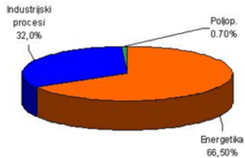
Sl. 4.5.: CO emisija iz ekonomskih sektora (42.99 Gg, 1990.)
