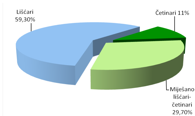
Slika 4.11.: Prikaz površina pod različitim tipovima sastojina šuma, u procentima.
