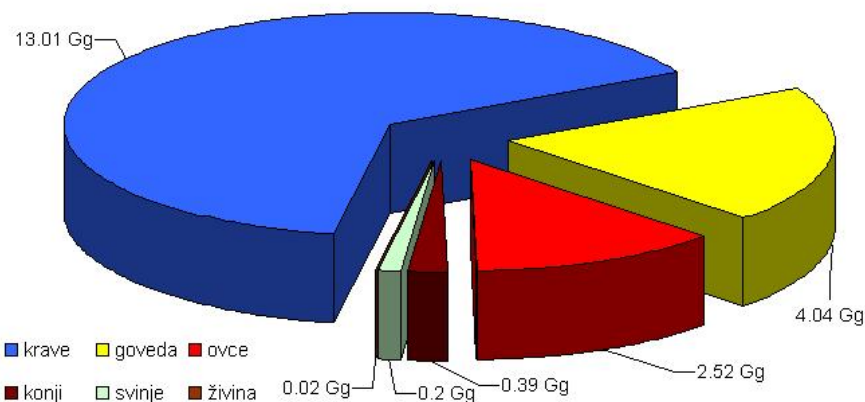
Slika 4.10.: CH 4 emisije usled enteričke fermentacije gajenih životinja u Crnoj Gori.
