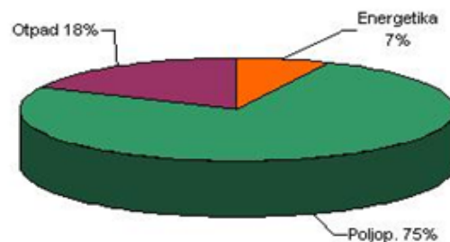
Sl. 4.2.: CH 4 emisija iz ekonomskih sektora (27.02 Gg, 1990.)
