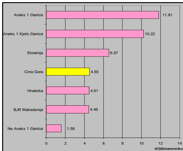
Slika 1.1.: Uporedne CO 2 emisije po stanovniku Crna Gora, zemlje iz regiona, Anex 1 i Ne-Anex 1 članice.
