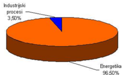
Sl. 4.7.: SO 2 emisija iz ekonomskih sektora (42.75 Gg, 1990.)
