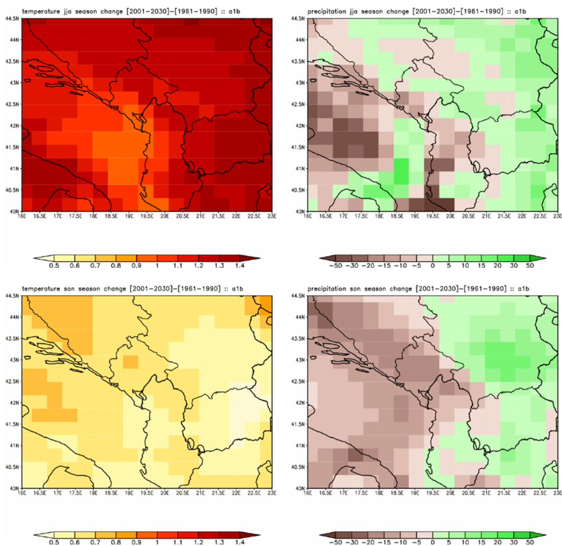
Slika 6.6: Promjene za JJA (gornji paneli) i SON (donji paneli) sezonu, temperature na 2 m (°C) (paneli levo) i akumuliranih padavina (%) (paneli desno) na teritoriji Crne Gore za A1B scenario tokom perioda 2001-2030.
