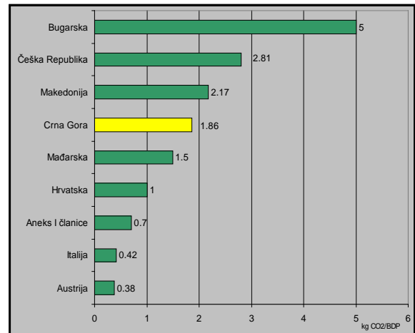
Slika 4.14.: Uporedne CO 2 emisije po kg CO 2 /USD po kursu iz 2000. godine, Crna Gora, zemlje iz regiona, Anex 1 članice (izvor podatak IEA, 2009)
