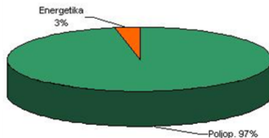
Sl. 4.3.: N 2 O emisija iz ekonomskih sektora (1.19 Gg, 1990.)
