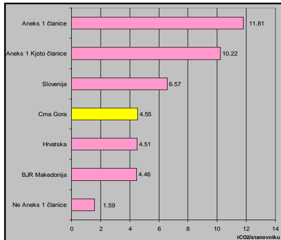
Slika 4.13.: Uporedne CO 2 emisije po stanovniku Crna Gora, zemlje iz regiona, Anex 1 i Ne-Anex 1 članice.
