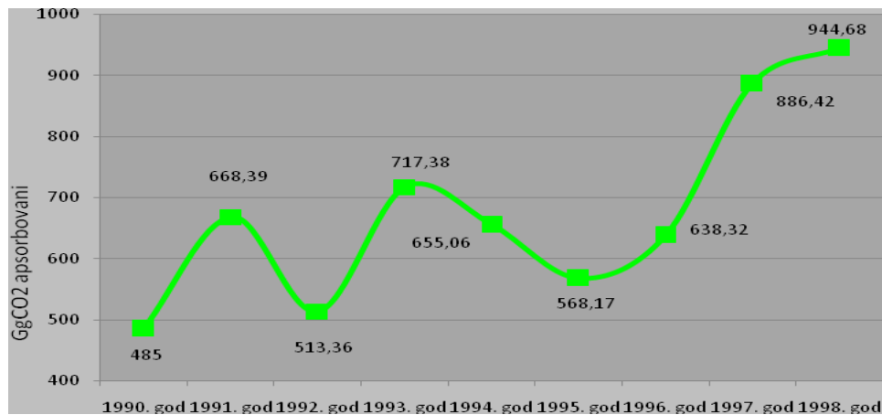
Slika 4.12.: Količina CO 2 u Gg apsorbovanog u ponorima.
