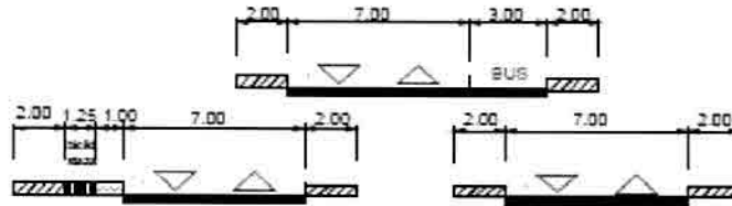
presjek 1-1
