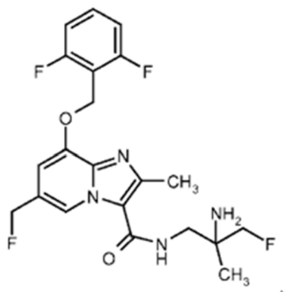
ent-N-(2-amino-3-fluoro-2-metilpropil)-8-[(2,6-difluorobenzil)oksi]-6-(fluorometil)-2-metilimidazo[1,2-a]piridin-3-karboksamid
