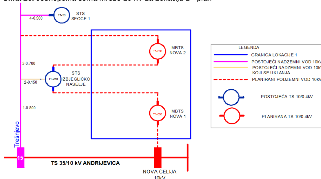
Slika 26. Jednopolna šema mreže 10 kV za Lokaciju 1 - plan
