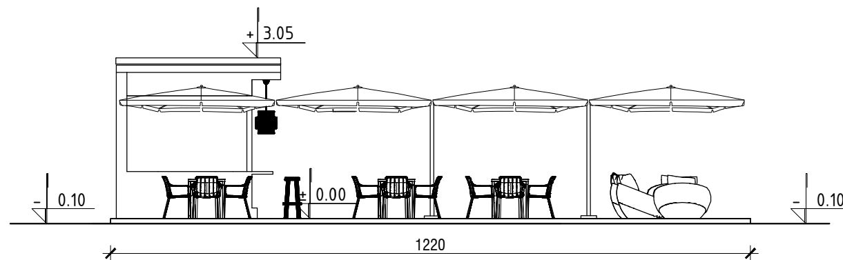
SEVEROZAPADNI IZGLED
