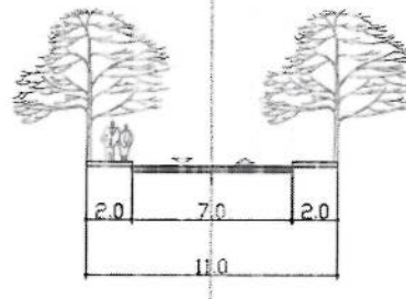
presjek 3-3
