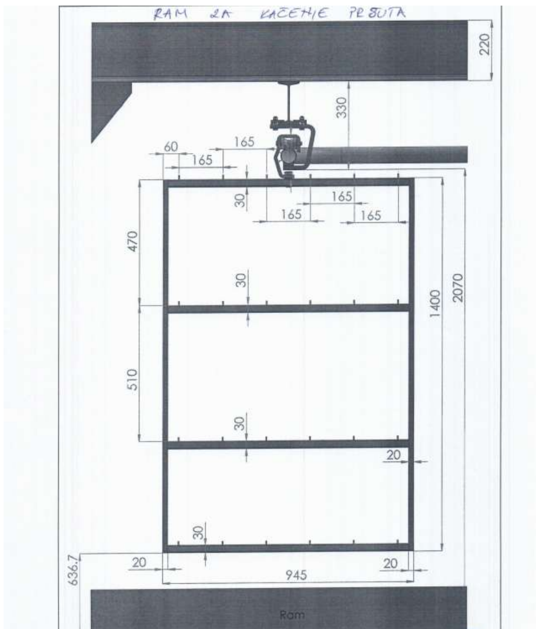
Skica 3 - Ramovi za kačenje pršuta sa kotrljajućom kukom
