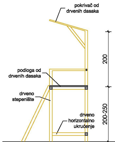
PRESJEK
