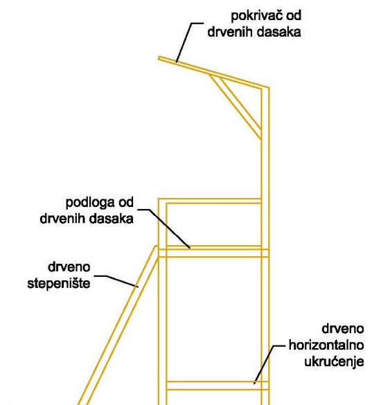
IZGLED A
