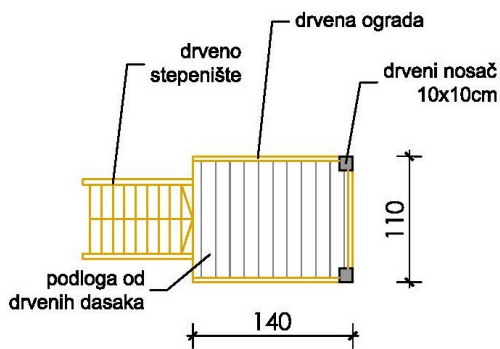
OSNOVA
