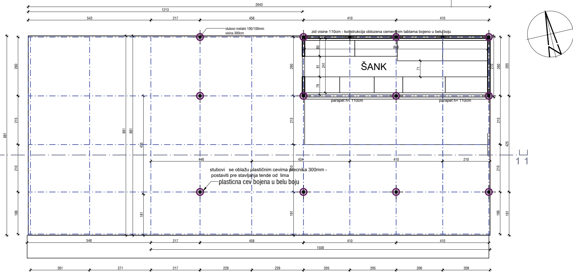
OSNOVA LOKALA SA PLANOM METALNE KONSTRUKCIJE ZA POSTAVLJANJE DEKINGA I POZICIJOM STUBOVA
