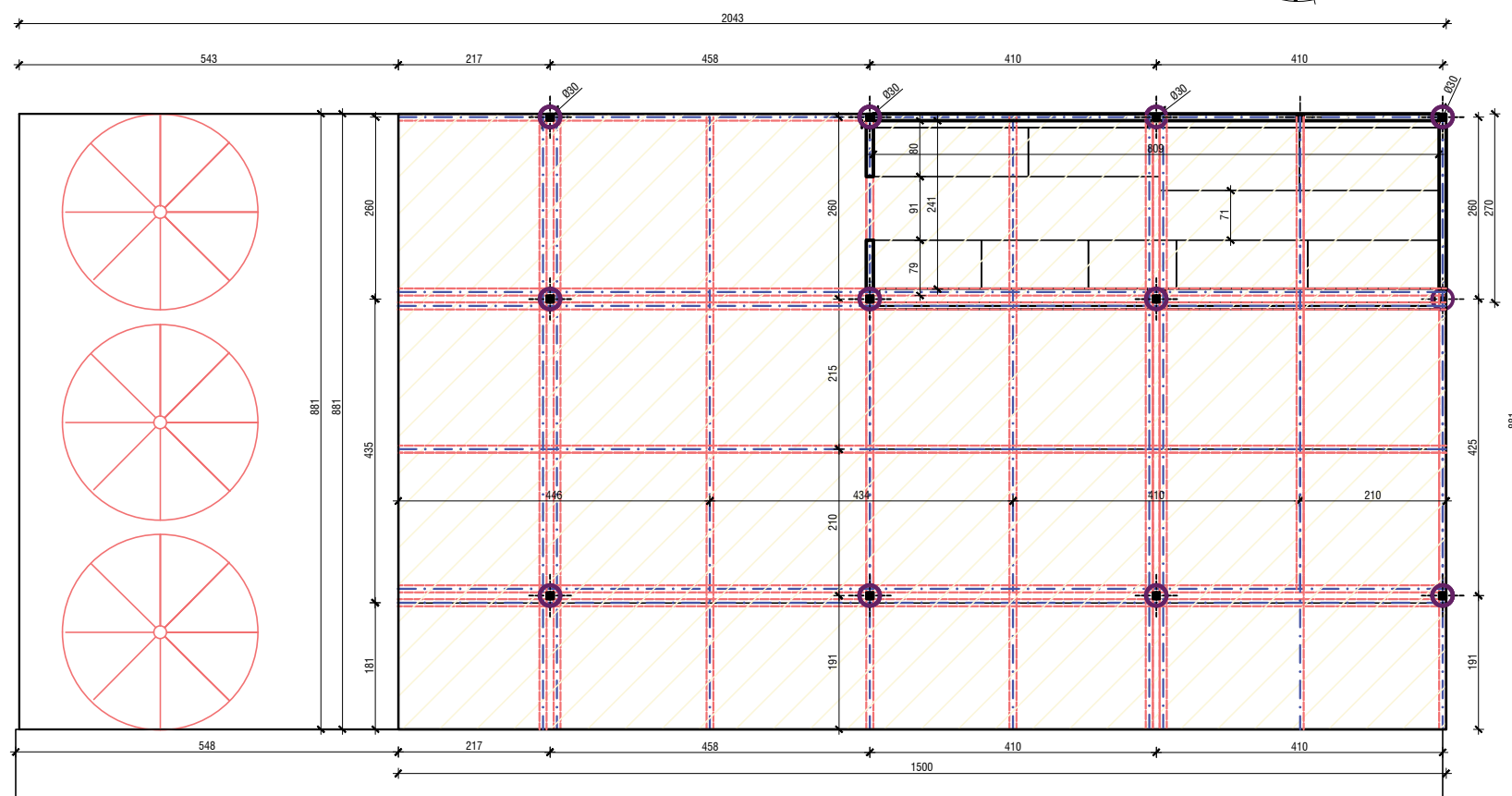
OSNOVA LOKALA SA PLANOM NADSTREŠNICE
