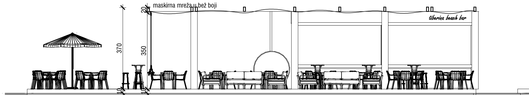
PRESEK 1-1
