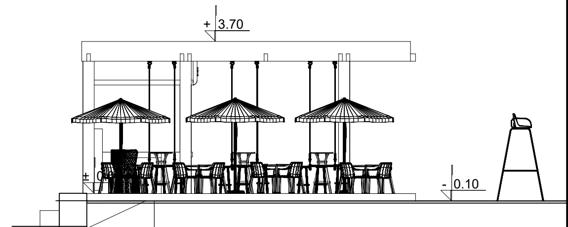
JUGOZAPADNI IZGLED
