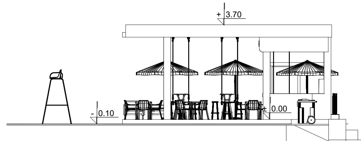
SEVEROISTOČNI IZGLED
