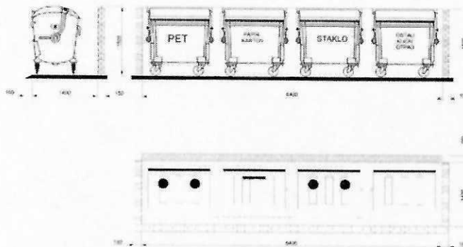
Dimenzije kontejnerskog boksa za 4 kontejnera kapaciteta 1,1\text{m}^3
