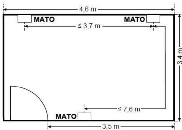
Slika 6: Primjer smještaja priključnih mjesta u prostoriji stana
