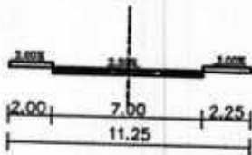
presjek B-B
