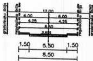
presjek D-D
