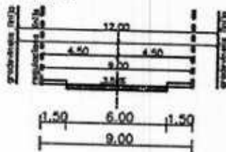
presjek C-C
