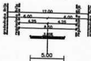
presjek G-G
