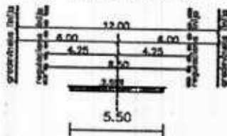
presjek E-E
