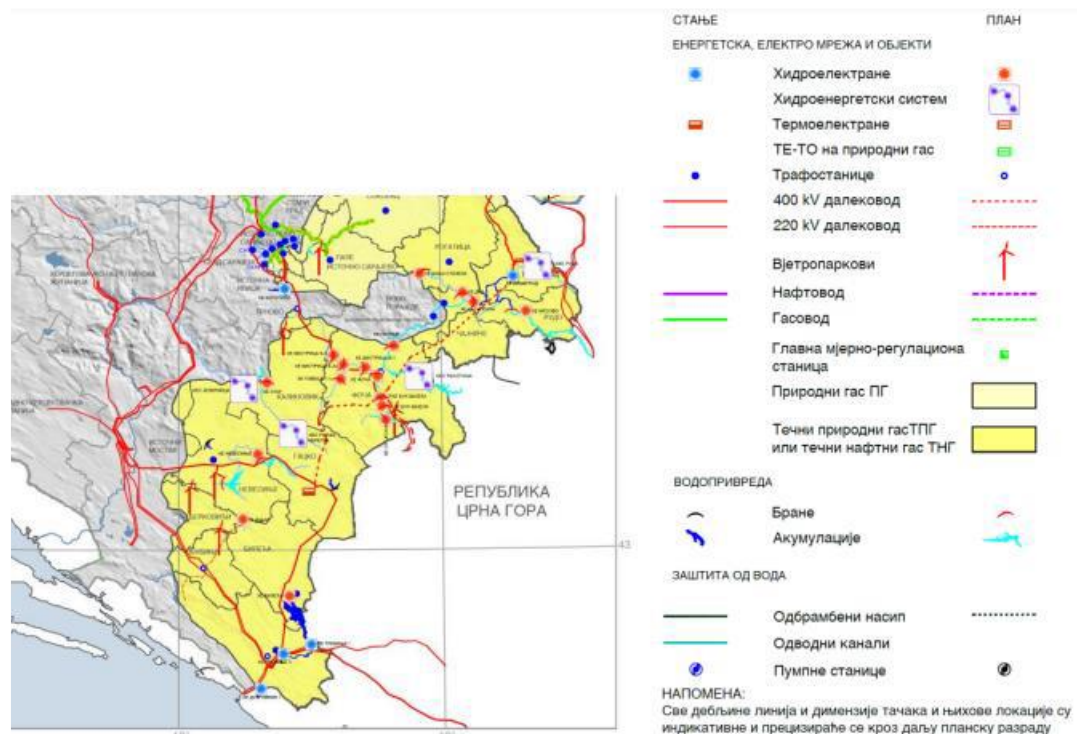
Slika 3. Izvod iz grafičkog dijela prostornog plana (Karta br. 21.4.1. Tehnička energetska infrastruktura, elektromreža i objekti).
