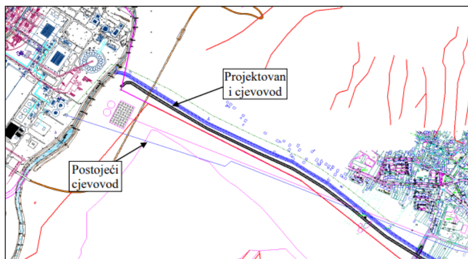
Slika 19. Izmještanje cjevovoda za snabdijevanje TE Gacko sirovom vodom (postojeća i nova trasa).
