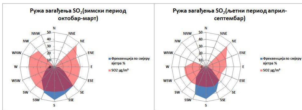
Grafikon 4. Ruže zagađenja \text{SO}_2 \mu\text{g}/\text{m}^3 Gacko M.M. krug O.Š. Sveti Sava 2021. godine https://rhmrzs.com/zivotna-sredina/kvalitet-vazduha/izvjestaj/godisnji-pregledi/
