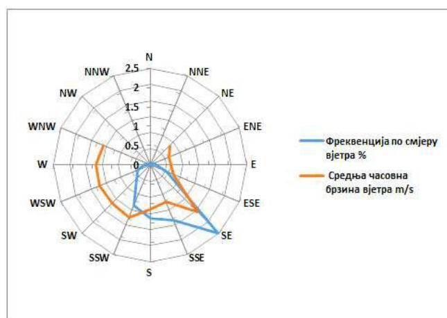
Slika 26 Prikaz čestine vjetra za mart 2024. u Gacku (mjernom mjestu krug OŠ „Sveti Sava“). (Izvod iz dokumenta Izvjestaju o kvalitetu vazduha u Republici Srpskoj za mjesec mart 2024. godine ).
