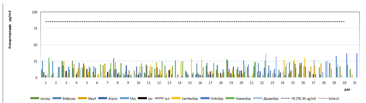
Dijagram 16: Grafički prikaz dnevne koncentracije NO 2 po danima za period januar – decembar 2021. godine u odnosu na granične vrijednosti (GV) i tolerantne vrijednosti (TV)
