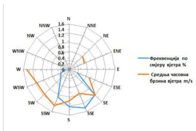
Slika 28. Prikaz čestine vjetra za maj 2024. u Gacku (mjernom mjestu krug OŠ „Sveti Sava“). (Izvod iz dokumenta Izvjештајu o kvalitetu vazduha u Republici Srpskoj za mjesec maj 2024. godine ).
