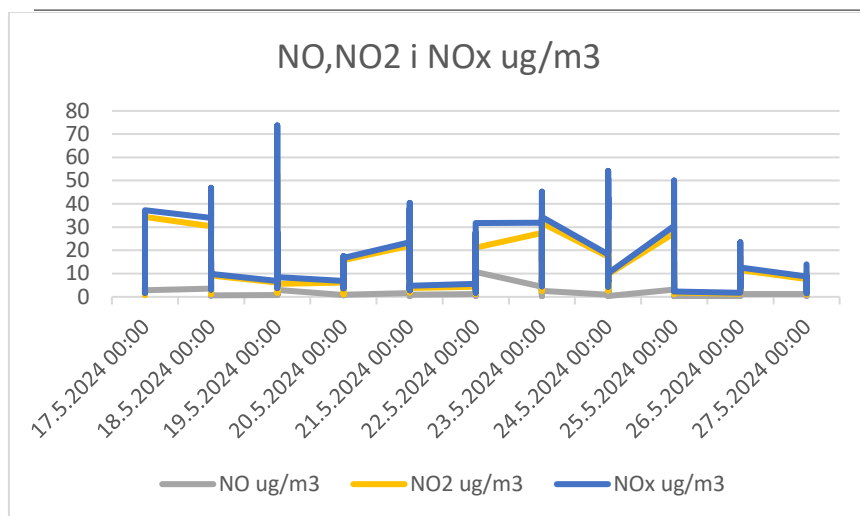
Slika 37. Grafički prikaz registrovanih imisionih koncentracija NO,NO 2 i NO x na lokaciji
