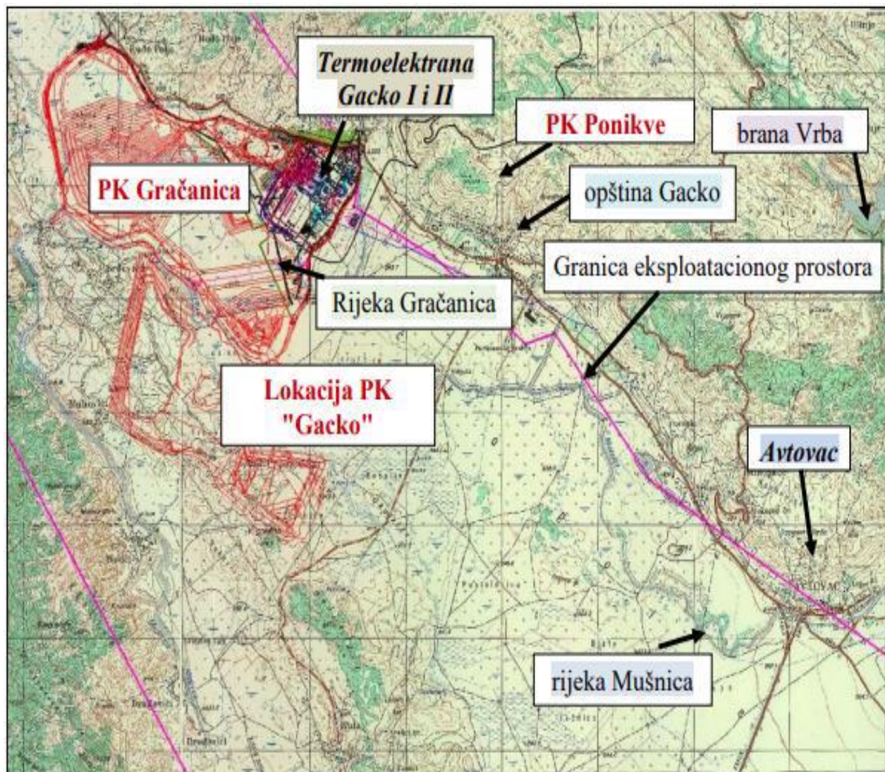
Slika 7. Prostorna lokacija Termoelektrana Gacko I i II i PK
