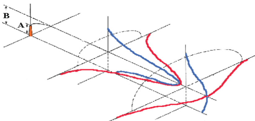
Slika 56. Raspodjela koncentracije prilikom kontinuiranog ispuštanja u atmosferu
