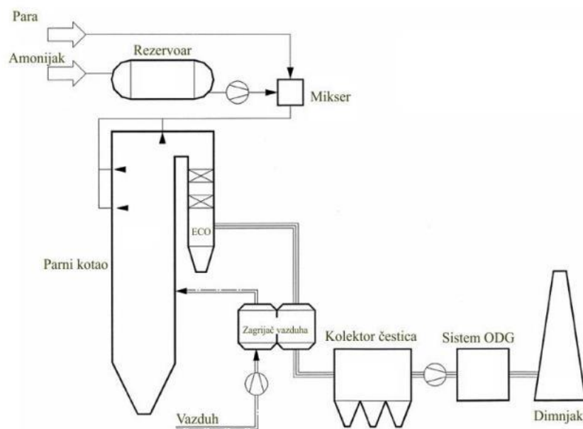
Slika 49. Procesni dijagram SNCR procesa.
