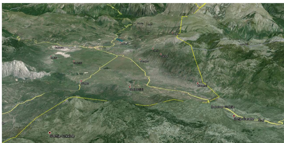
Slika 12. Izgled Gatačkog karsnog polja
