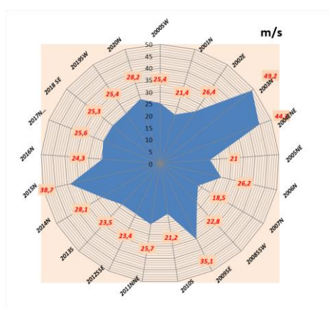
Slika 23. Maksimalna brzina vjetra za period 2000.-2020. godine (meteorološke stanice RiTE Gacko).
