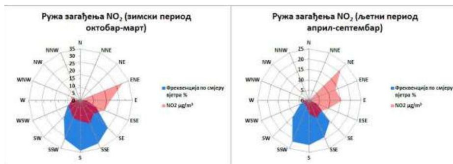
Grafikon 17. Ruže zagađenja \text{NO}_2 \mu\text{g}/\text{m}^3 Gacko M.M. krug O.Š. Sveti Sava 2023
