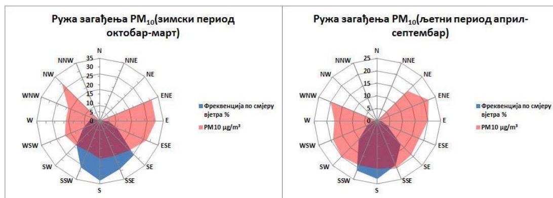
Grafikon 6. Ruže zagađenja PM10 \mu\text{g}/\text{m}^3 Gacko M.M. krug O.Š. "Sveti Sava" 2021. godine https://rhmrzs.com/zivotna-sredina/kvalitet-vazduha/izvjestaj/godisnji-pregledi/
