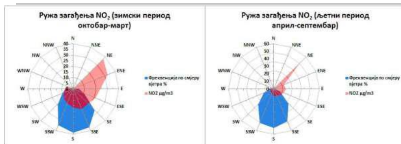
Grafikon 12. Ruže zagađenja \text{NO}_2 \mu\text{g}/\text{m}^3 Gacko M.M. krug O.Š. Sveti Sava 2022. godine https://rhmrzs.com/zivotna-sredina/kvalitet-vazduha/izvjestaj/godisnji-pregledi/
