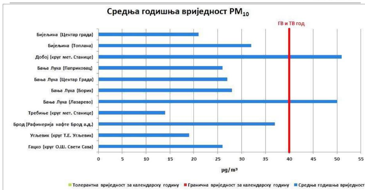
Графикон 13. Упоредни приказ средње годишње концентрације PM 10 µg/m³ по мјерним мјестима у 2022. години
