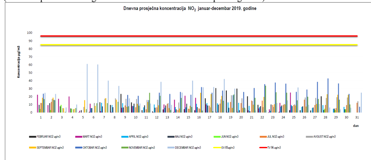
Dijagram 4: Grafički prikaz dnevne prosječne koncentracija NO 2 za period januar – decembar 2019. godine po danima u odnosu na dnevnu graničnu vrijednost (GV) i tolerantnu vrijednost (TV)
