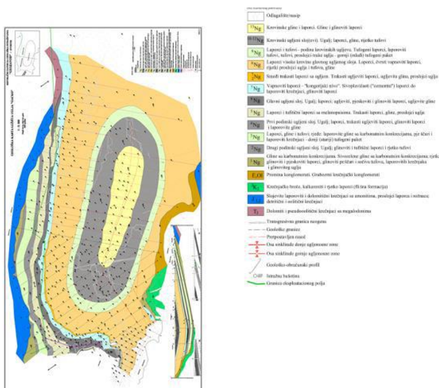
Slika 11. Pregledna geološka karta šireg područja Gacka
