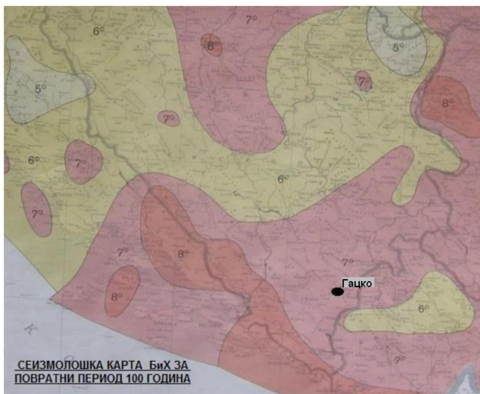
Slika 15. Položaj Gacka na seizmološkoj karti za povratni period od 100 godina
