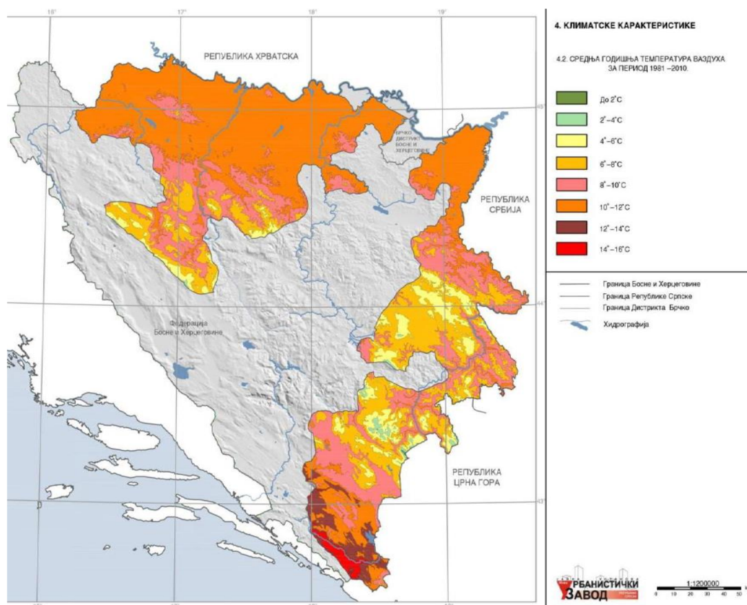
Slika 20. Srednja godišnja temperatura vazduha za period 1981-2010 (Izvod iz dokumenta Izmjene i dopune Prostornog plana Republike Srpske do 2025. godine).
