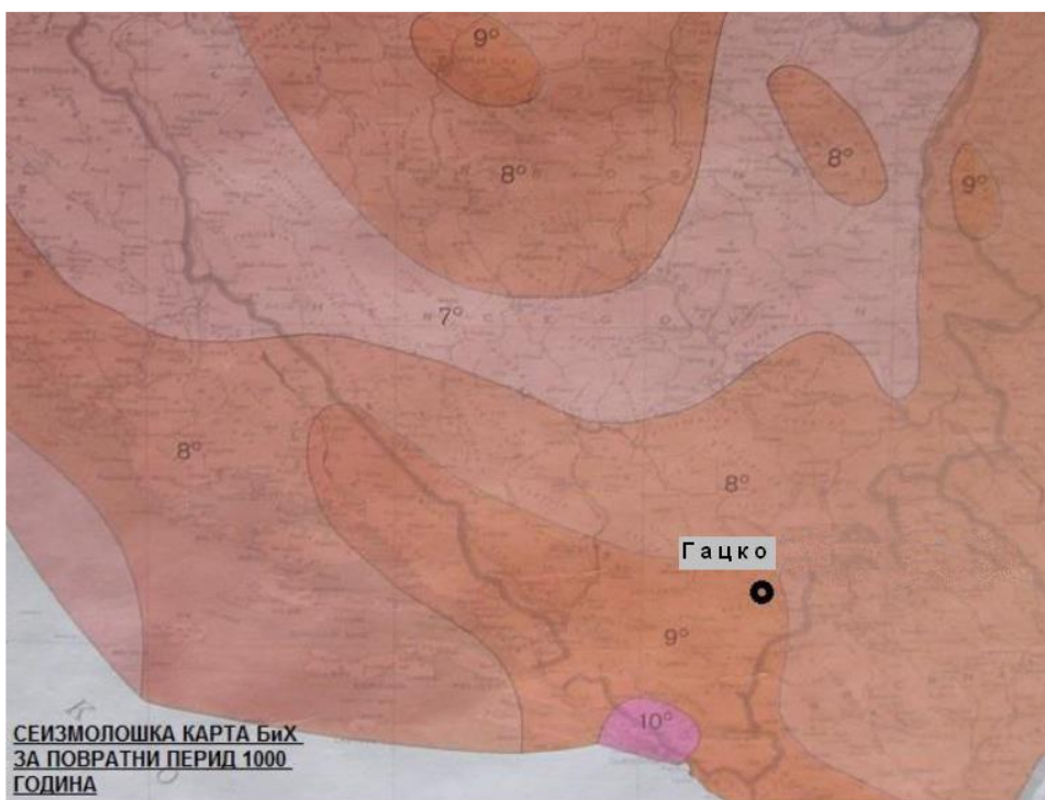
Slika 16. Položaj Gacka na seizmološkoj karti za povratni period od 1000 godina
