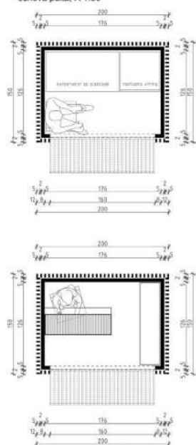
osnova pulta, R 1:50
