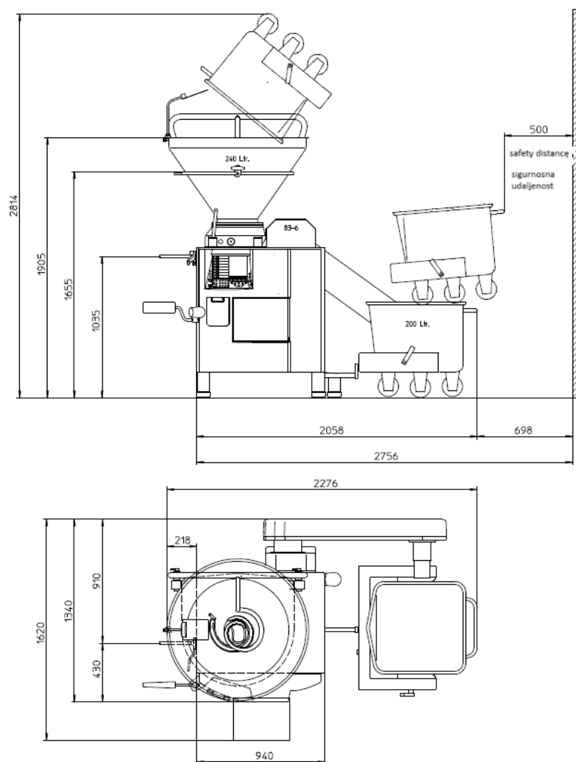
Skica 1 - Lift za kuter kolica
