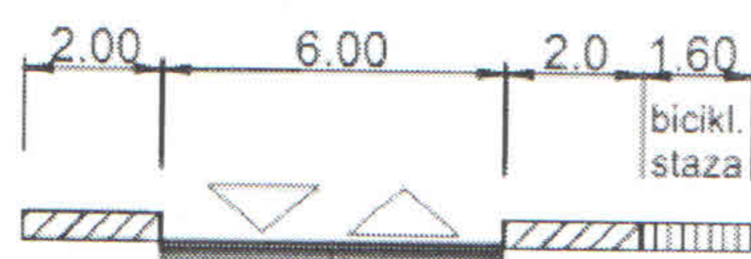
presjek 2-2
