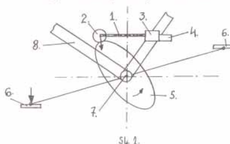
Uređaj za akumuliranje obrtnog momenta kod bicikla
