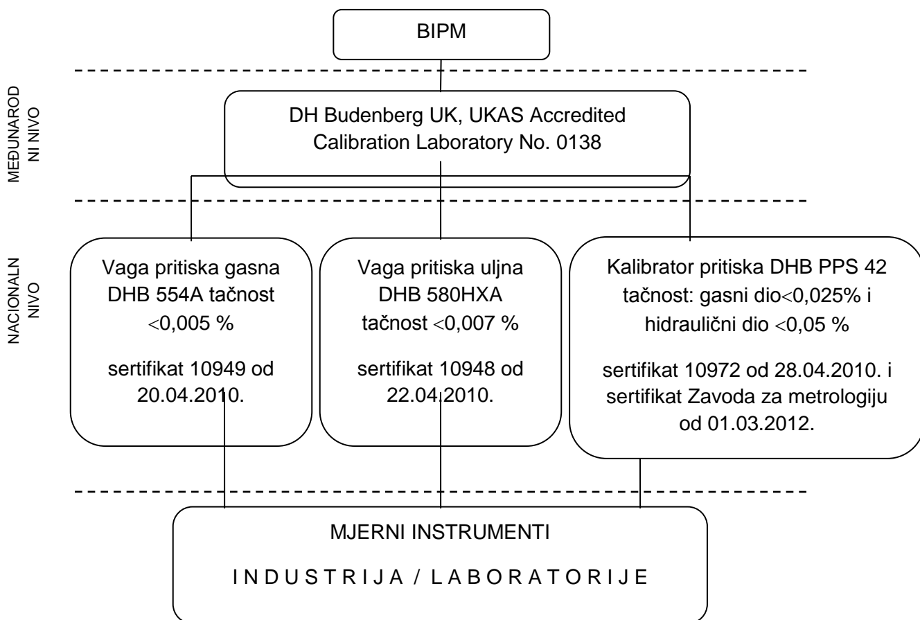
Slika 4. Lanac sljedivosti u oblasti mjerenja pritiska
