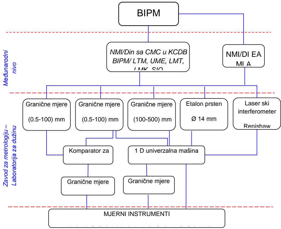
Slika 2. Lanac sljedivosti u oblasti mjerenja dužine
