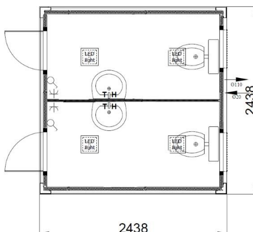
SANITARNI KONTEJNER TIP „EUROmodul“ standard MODEL 1173
