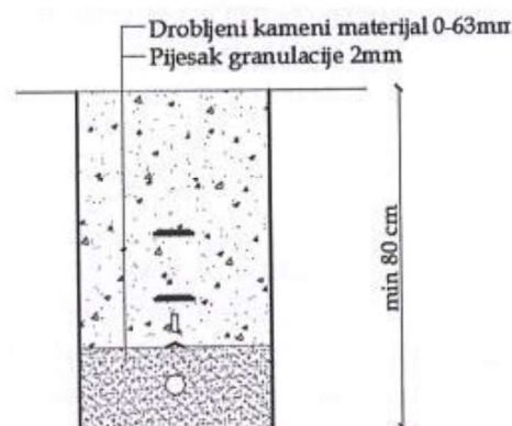
sl. 2 - Detalj rova za polaganje kablova u zoni bankine
