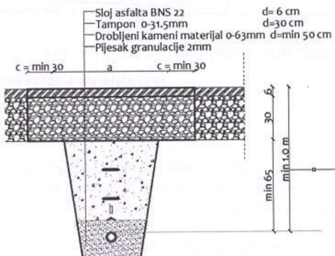
sl. 1 - Detalj rova za polaganje kablova u zoni kolovoza sa asfaltnim zastorom
