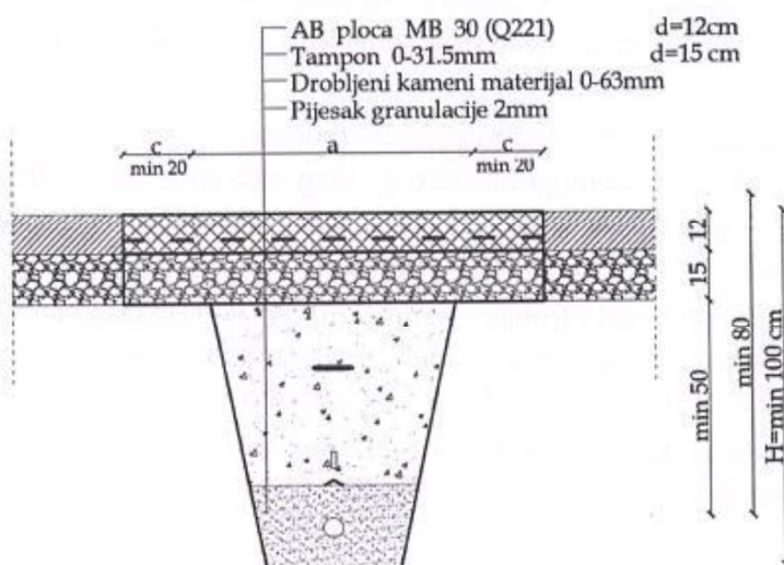
sl. 3 - Detalj rova za polaganje kablova u zoni trotoara
