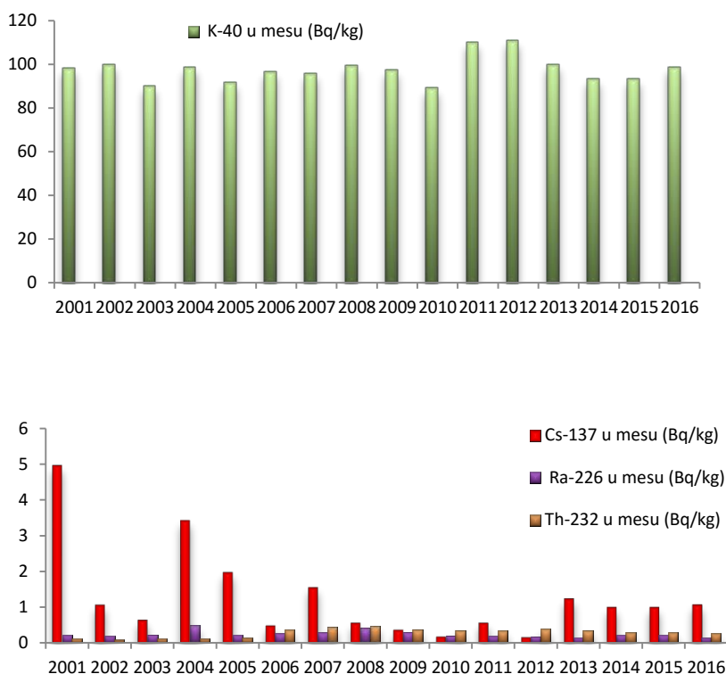
Grafikon 106. Specifične aktivnosti radionuklida u goveđem i jagnječem mesu, u periodu 2001-2016. godine, izvedene analizom uzoraka sa cijele teritorije Crne Gore. Specifične aktivnosti kalijuma ^{40}\text{K} su prikazane odvojeno (gornji grafik na slici).
