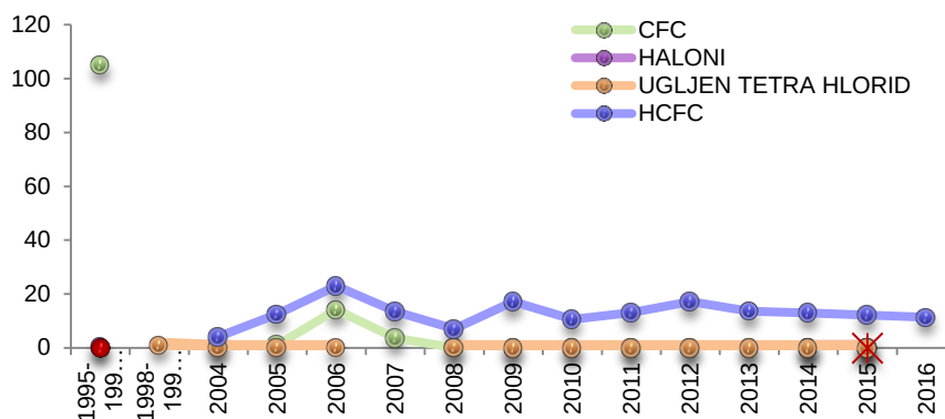
Grafikon 28. Potrošnja supstanci koje oštećuju ozonski omotač, 1995 -2016. (t)
