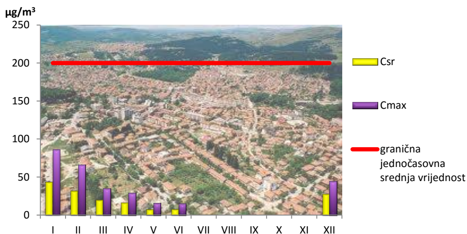
Grafikon 14. Koncentracija \text{NO}_2 u vazduhu- Pljevlja
