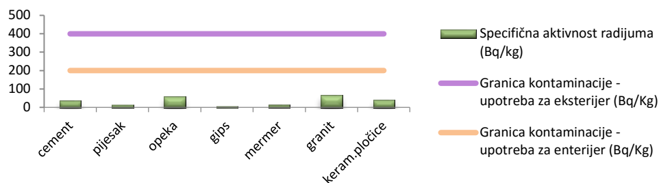
Grafikon 102. Specifične aktivnosti ^{226}\text{Ra} (Bq/kg) izvedene iz analiziranih uzoraka građevinskih materijala na teritoriji Crne Gore u 2016. godini u poređenju sa maksimalno dozvoljenim granicama.
