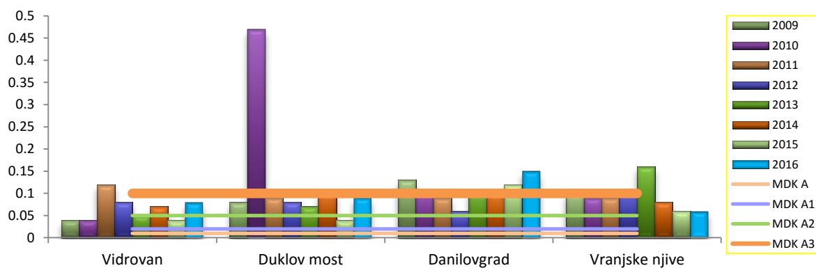
Grafikon 37. Sadržaj ortofosfata(fosfata) u rijeci Zeti (mg/l)
