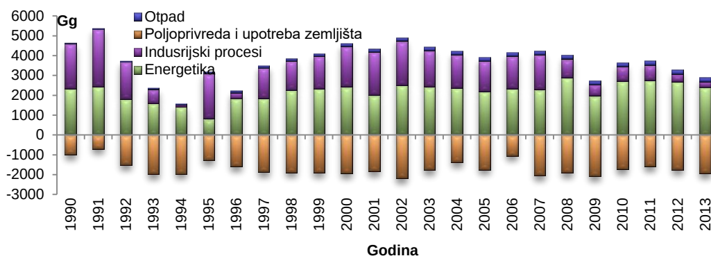
Grafikon 18. GHG emisije izražene kao CO 2 eq po sektorima, 1990-2013. (Gg)
