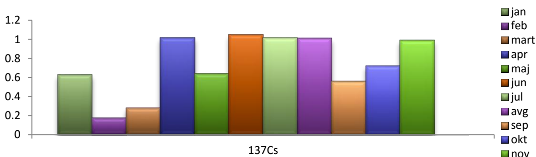
Grafikon 101. Koncentracije aktivnosti radionuklida ^{137}\text{Cs} u mjesečnim uzorcima padavina, izražene u mBq/l za 2016. godinu.
