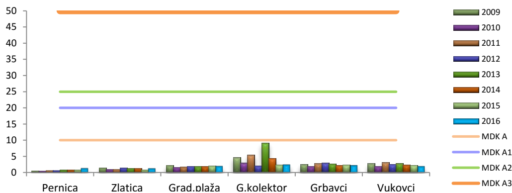
Grafikon 41. Sadržaj nitrata u rijeci Morači (mg/l)
