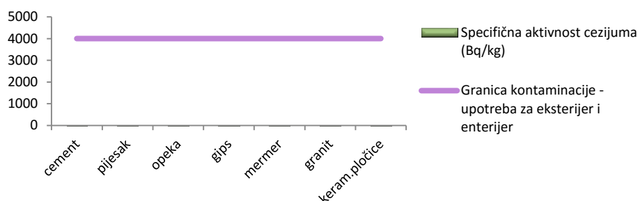
Grafikon 105. Specifične aktivnosti ^{137}\text{Cs} (Bq/kg) izvedene iz analiziranih uzoraka građevinskih materijala na teritoriji Crne Gore u 2016. godini u poređenju sa maksimalno dozvoljenim granicama.
