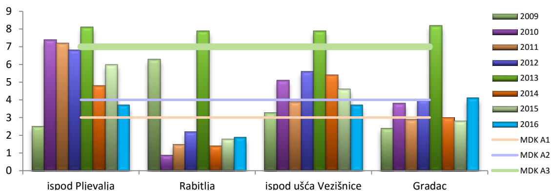
Grafikon 33. BPK_5 u rijeci Čehotini (mg/l)
