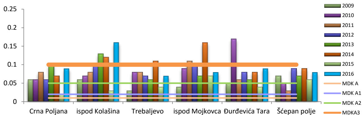
Grafikon 36. Sadržaj ortofosfata(fosfata) u rijeci Tari (mg/l)
