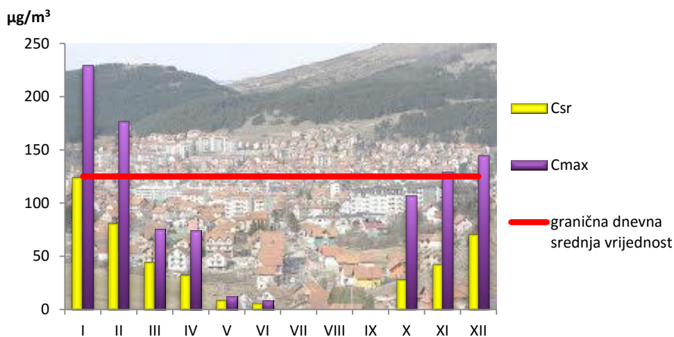
Grafikon 13. Koncentracija \text{SO}_2 u vazduhu-Pljevlja
