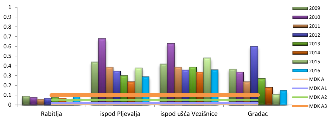
Grafikon 38. Sadržaj ortofosfata (fosfata) u rijeci Ćehotini (mg/l)
