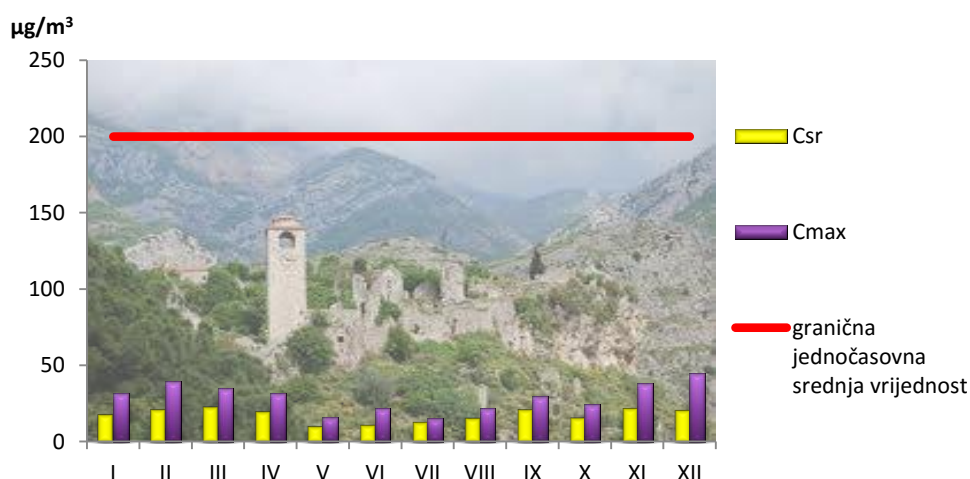
Grafikon 5. Koncentracija \text{NO}_2 u vazduhu-Bar
