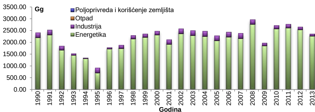
Grafikon 19. Ukupne emisije CO 2 po sektorima, 1990-2013. (Gg)
