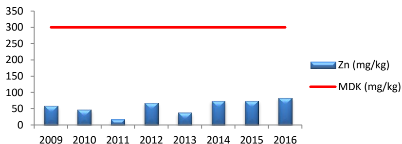
Grafikon 65. Sadržaj cinka (Zn) u uzorku zemljišta uzorkovanom na obali Crnog jezera, 2009-2016
