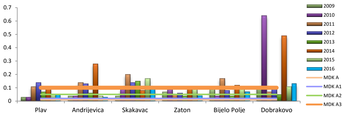
Grafikon 39. Sadržaj ortofosfata(fosfata) u rijeci Lim (mg/l)
