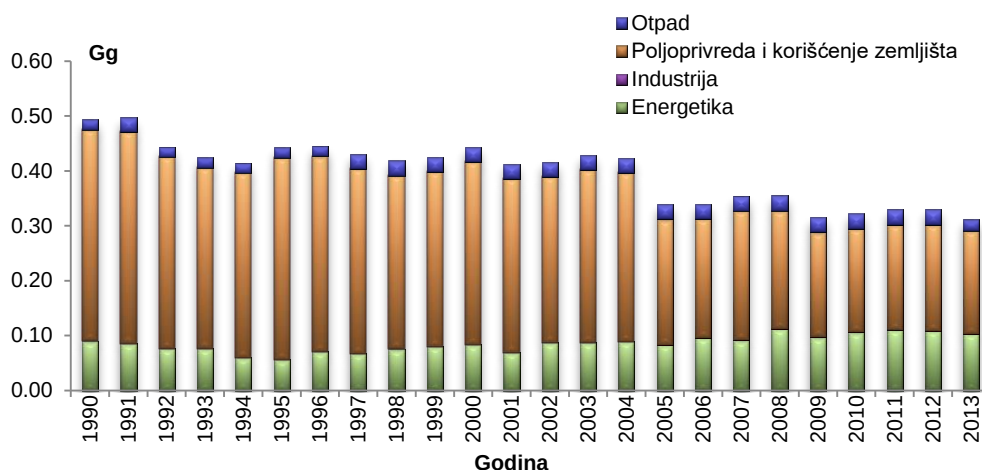
Grafikon 22. Ukupne emisije N_2O po sektorima, 1990-2013. (Gg)
