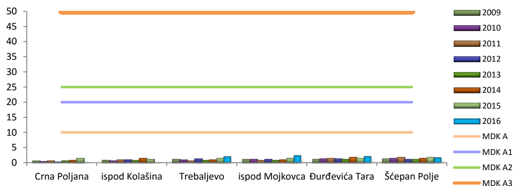
Grafikon 44. Sadržaj nitrata u rijeci Tari (mg/l)
