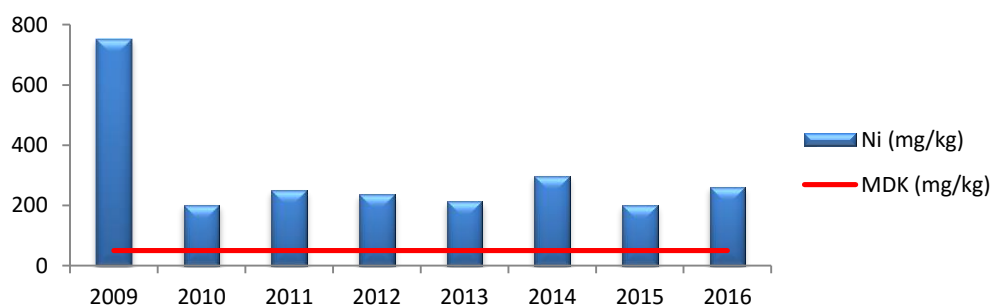
Grafikon 83. Sadržaj nikla (Ni) u uzorku zemljišta uzorkovanom na Ulcinjskom polju, 2009-2016
