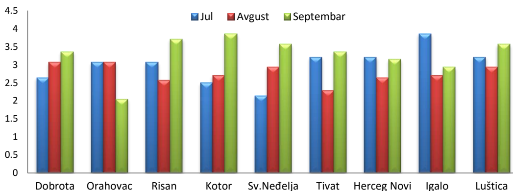
Grafikon 55. Koncentracija nitrata ( \mu\text{mol/l} ) na pozicijama u Bokotorskom zalivu
