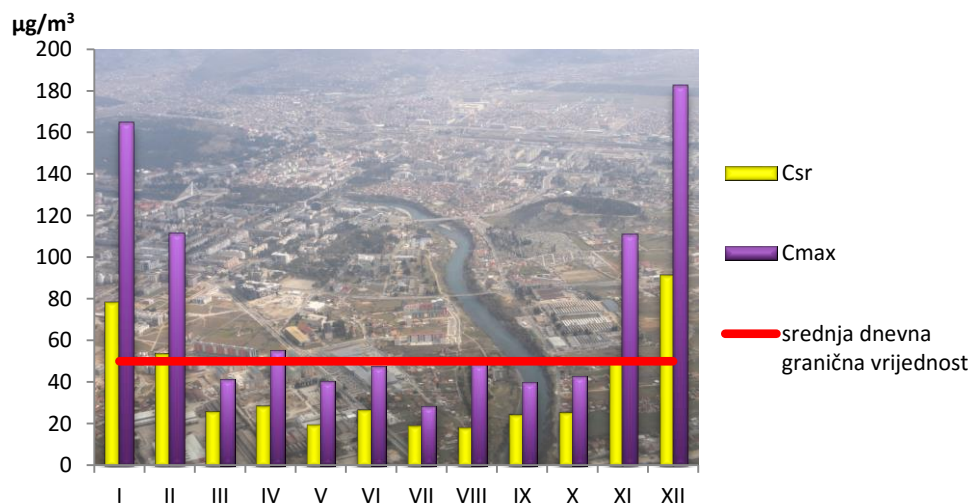
Grafikon 3. Koncentracija PM 10 u vazduhu-Podgorica
