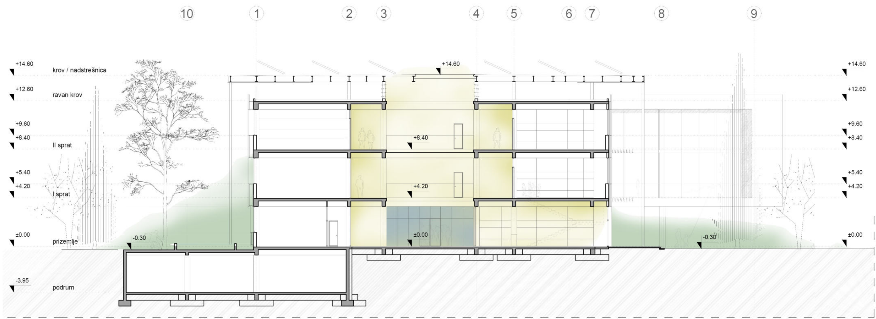
PRESJEK 2-2 R=1:200
