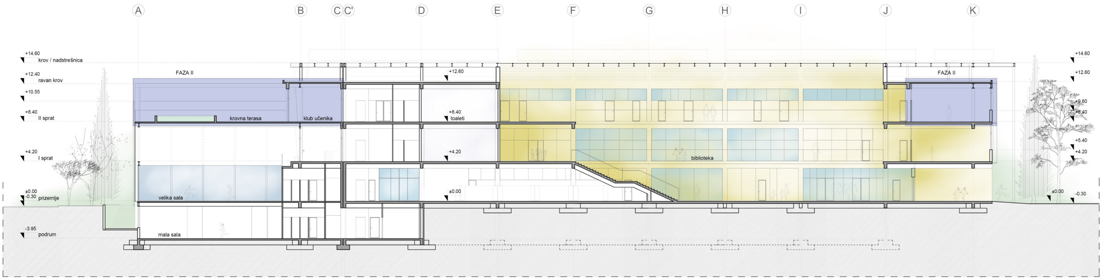
PRESJEK 1-1 R=1:200
