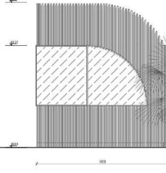
pogled 2, R 1:50
