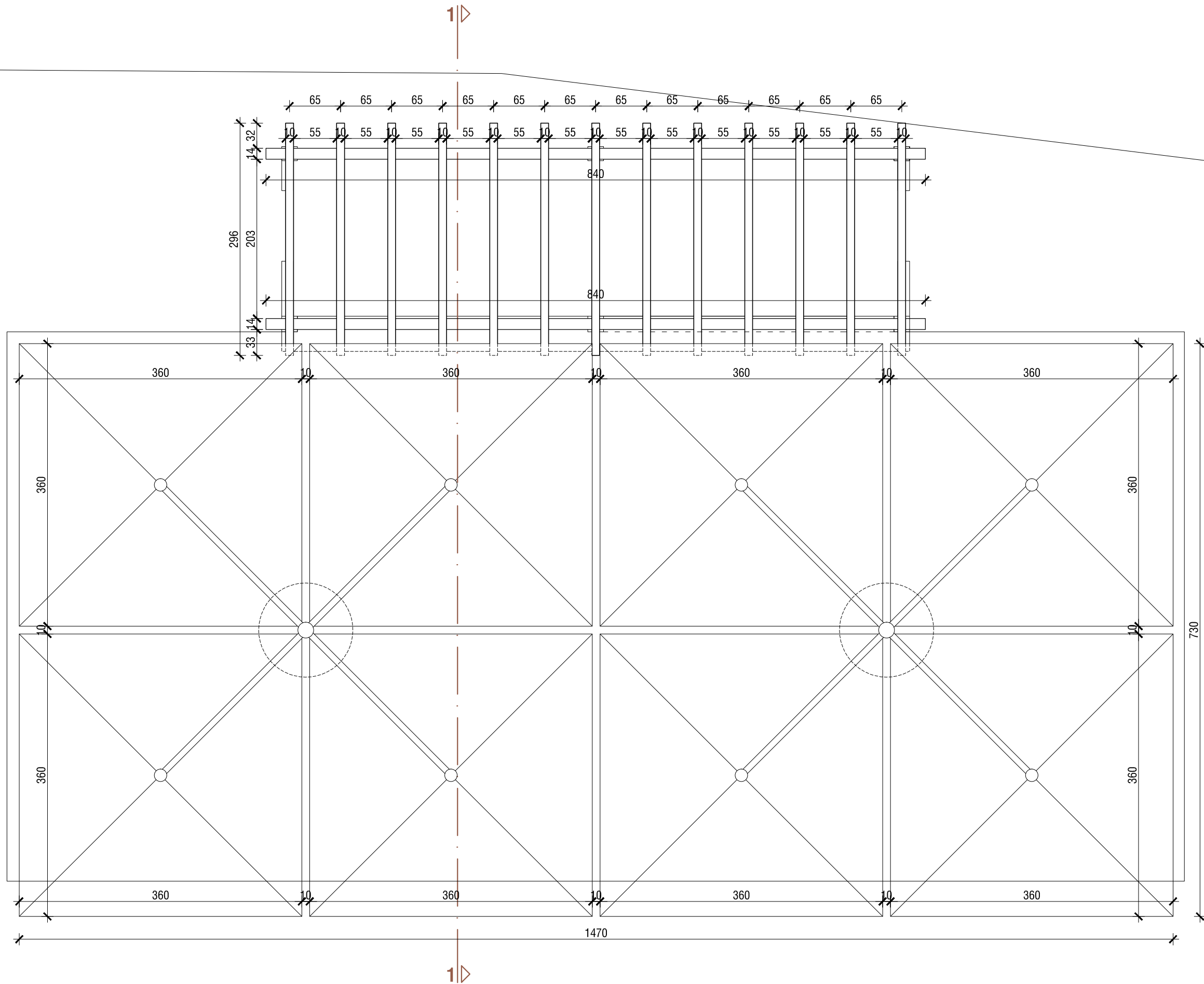
DRVENA KROVNA KONSTRUKCIJA NADSTREŠNICE ŠANKA I SUNCOBRA NA TERASI
