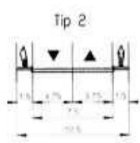
PRESJEK B __ B
