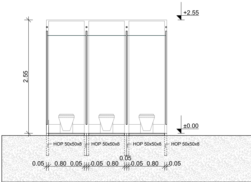
PRESJEK 1-1
