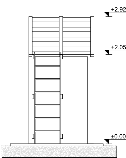
IZGLED 4
