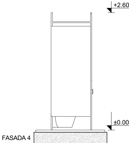
FASADA 4
