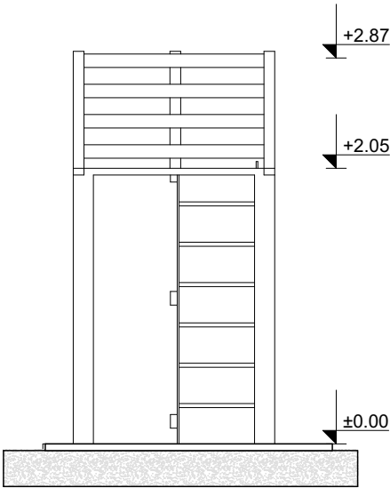
IZGLED 3
