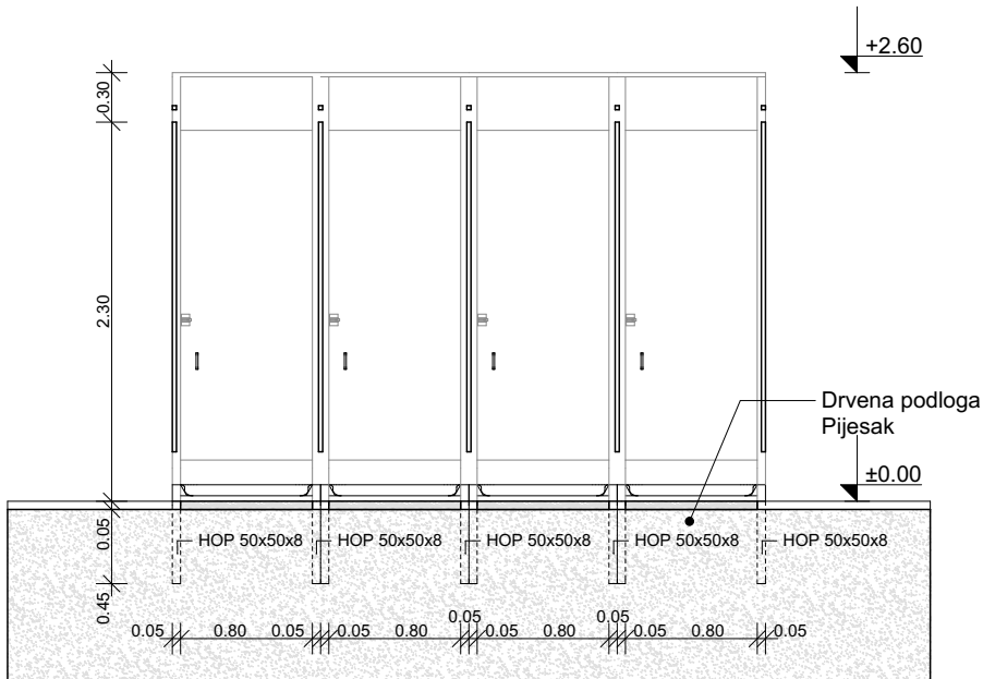
PRESJEK 1-1
