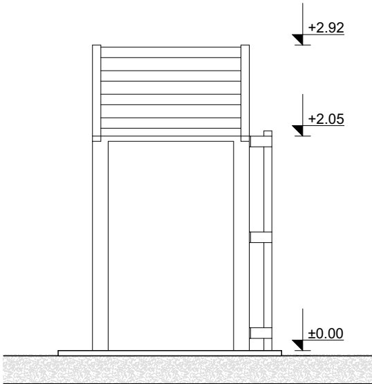
IZGLED 1
