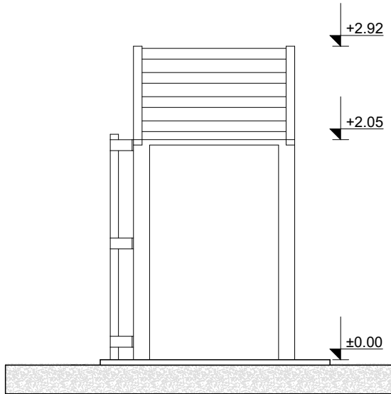
IZGLED 2
