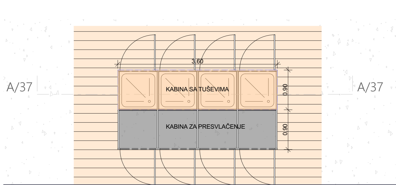
OSNOVA
